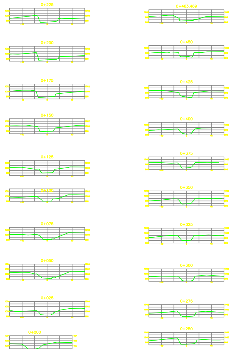
SECCIONES DE RIO QUILICHAO AGUAS ABAJO
