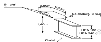
DETALLE B PUNTA DEL CODAL
