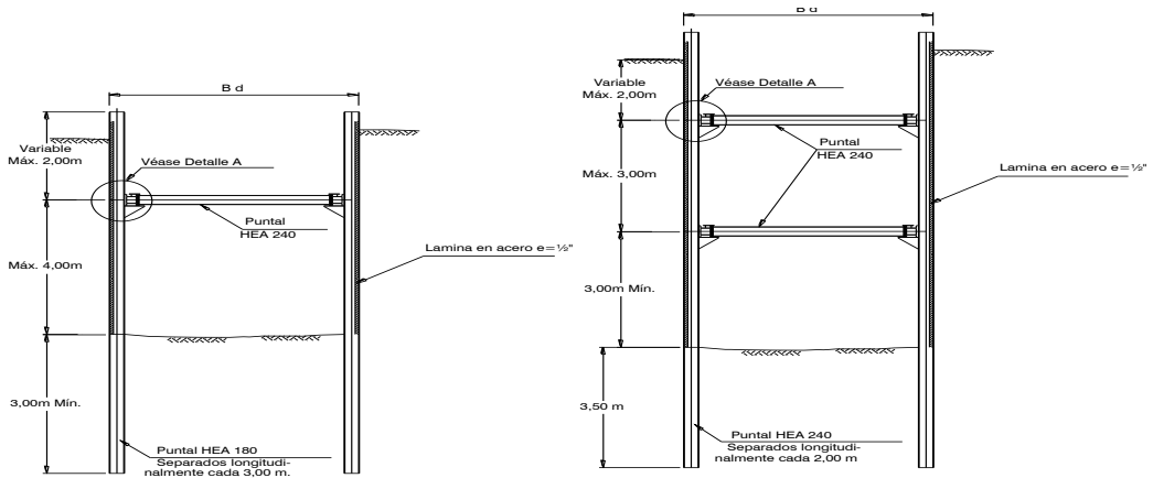
PARA PROFUNDIDADES DE 6.00 A 8.00 METROS
