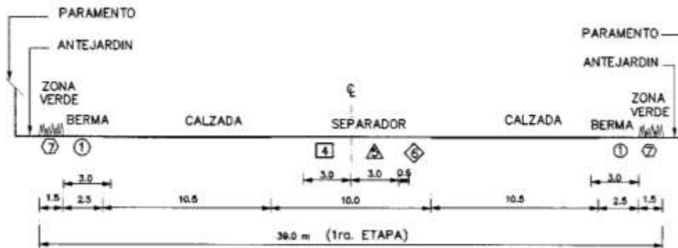
Esquema 23. Localización de redes de servicios en las vías
