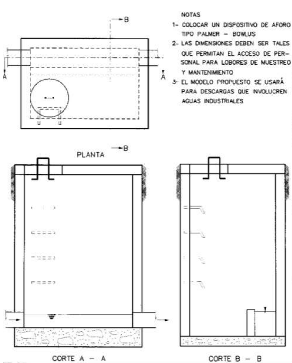
Esquema 62. Cámara de inspección para muestreo y aforo de aguas industriales
