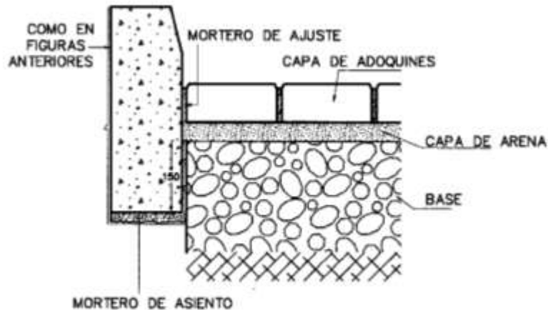
g. profundidad de empotramiento en pavimentos de adoquines.
