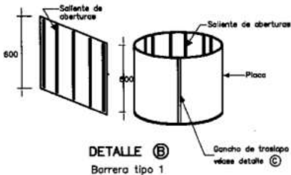
Esquema 8. Barrera Trapezoidal para Control Radicular
