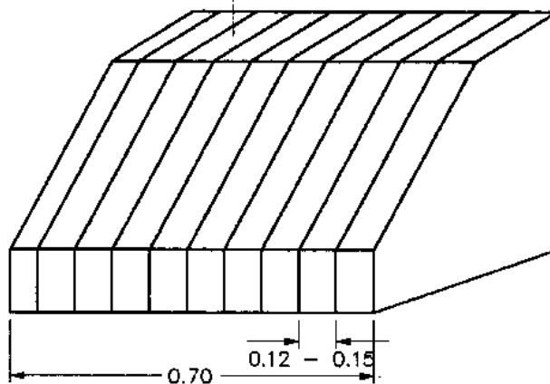
DISTRIBUCION DE FRANJAS AMARILLAS Y NEGRAS
