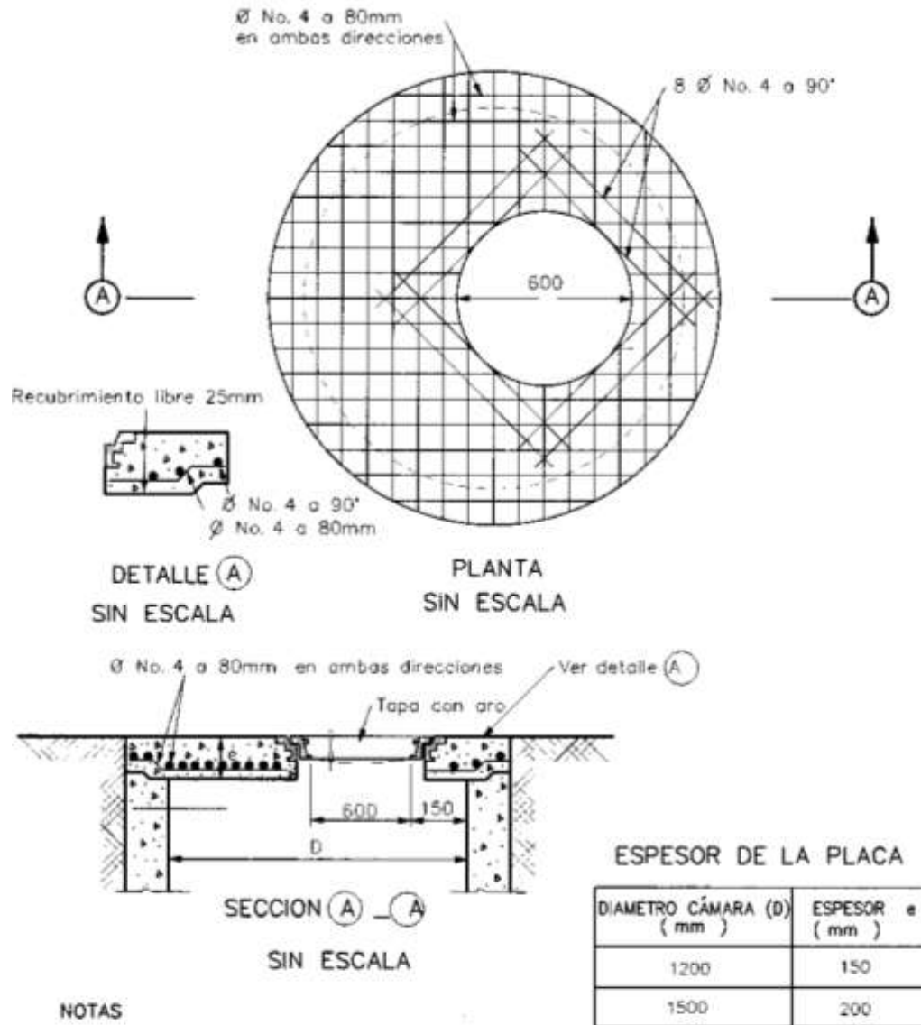
Esquema 50. Placa de superficie para cámara de inspección
