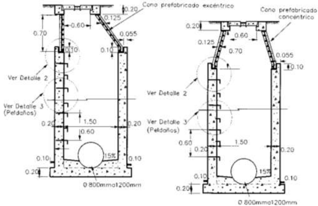
CÁMARA EXCÉNTRICA
