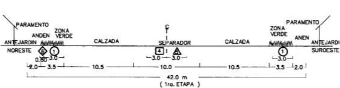
Esquema 43. Localización de Redes de Servicios en las Vías
