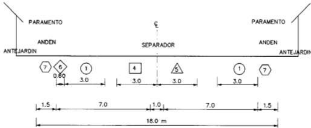
Esquema 35. Localización de Redes de Servicios en las Vías
