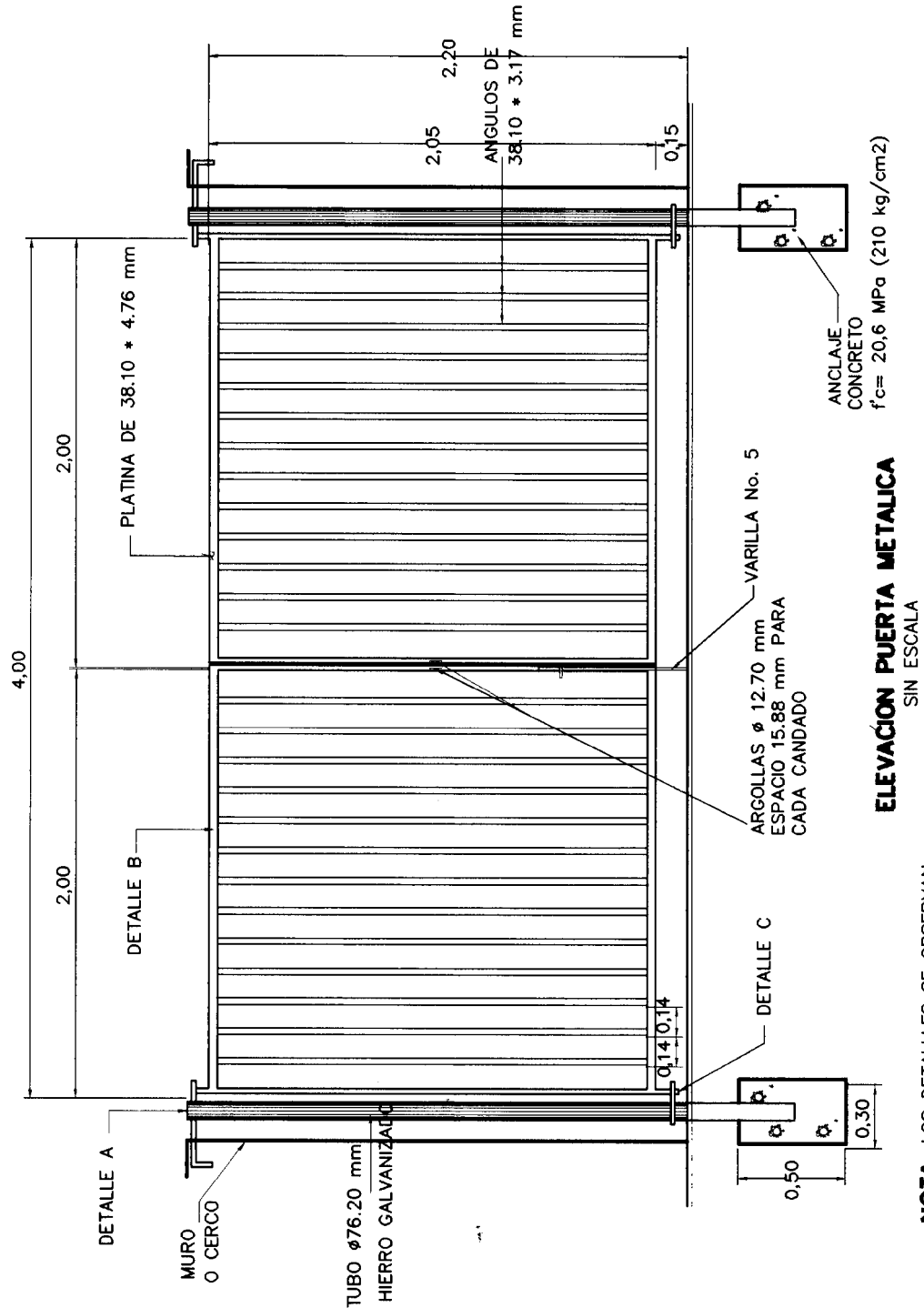
Esquema 14. Detalles Puerta Metálica
