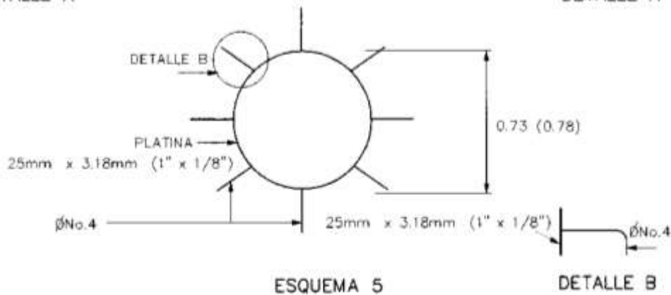
ESQUEMA 5 HERRAJE DEL CUELLO PARA REALCE DE 2.5 A 6.1 CM.
