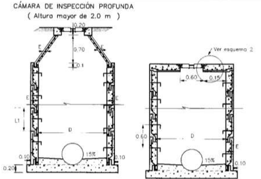
CÁMARA DE INSPECCIÓN DE Poca PROFUNDIDAD ( Altura menor de 2.0 m )
