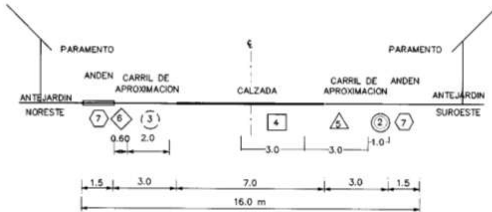
Esquema 36. Localización de Redes de Servicios en las Vías
