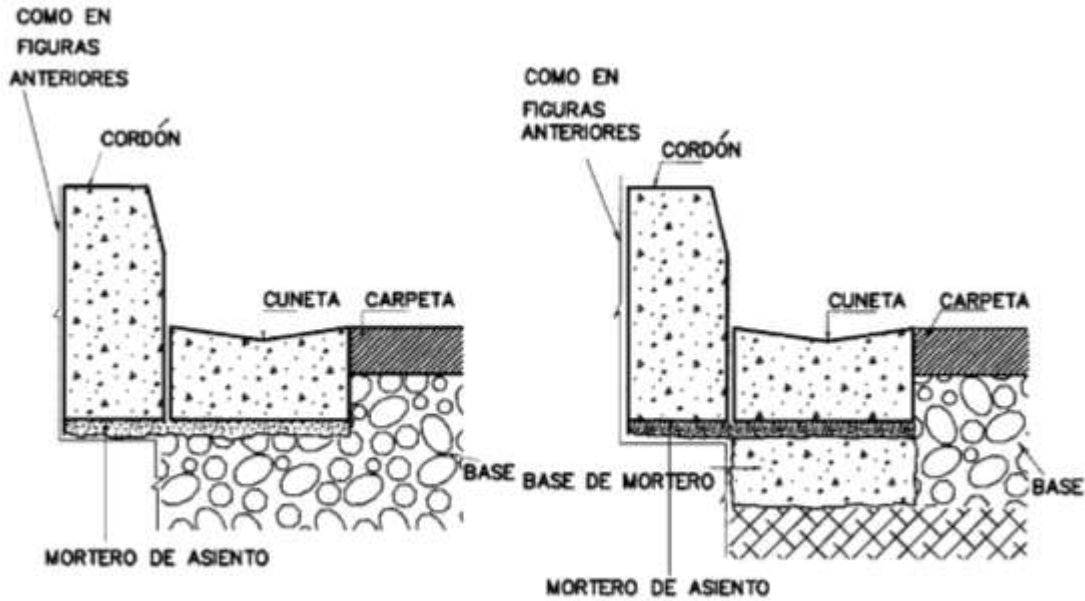
e. cunetas sobre base del pavimento.
