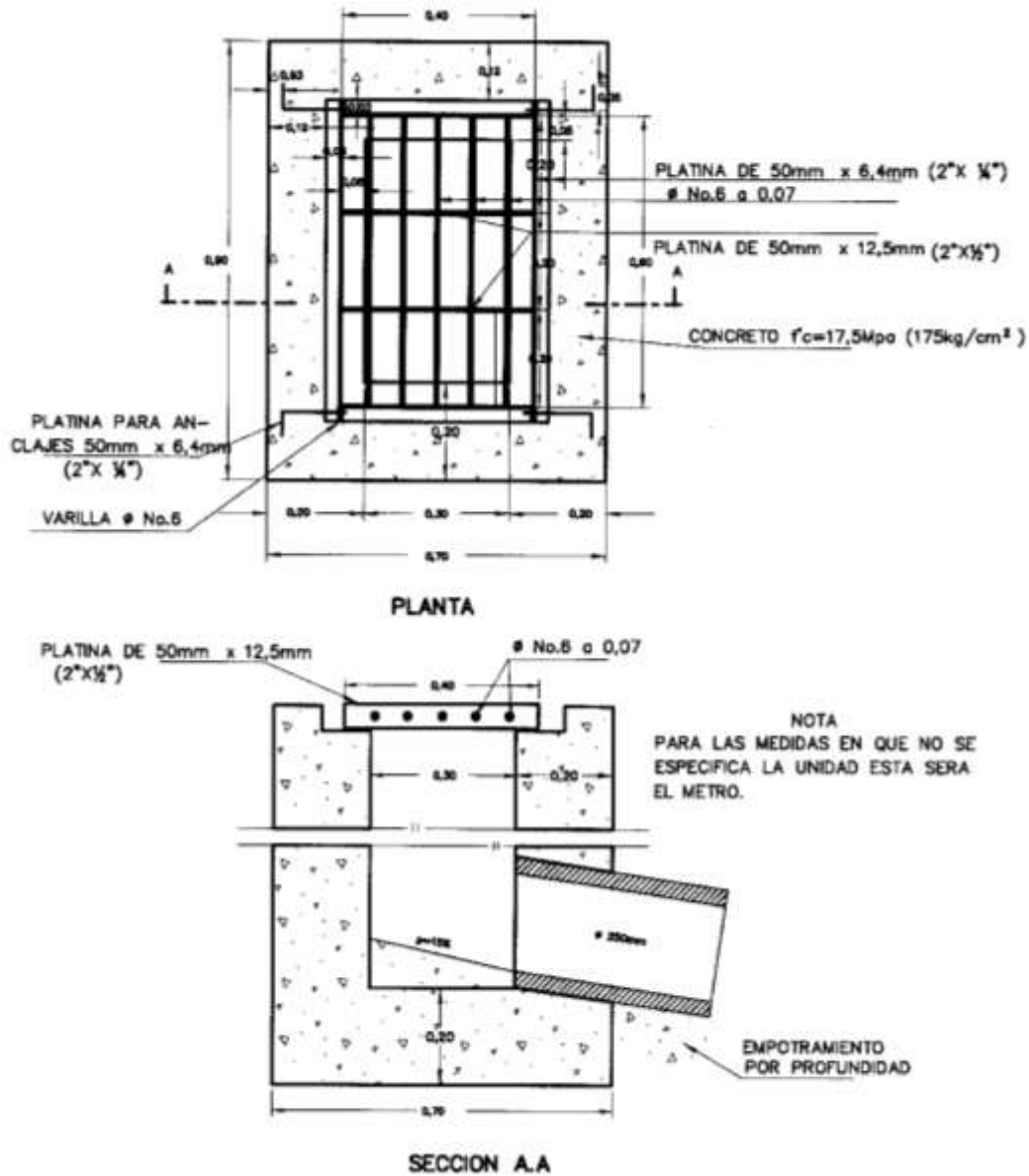
Esquema 67. Sumidero de aguas lluvias TIPO A
