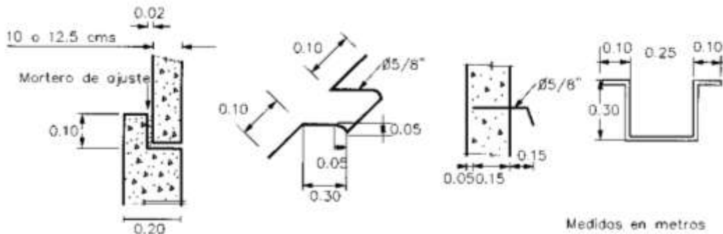
DETALLE 1 Apoyo de cono
