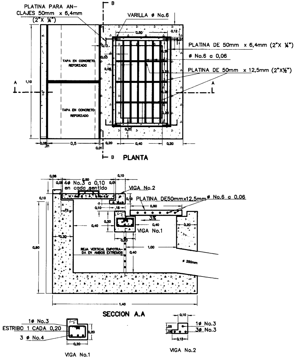
Esquema 69. Sumidero de Captación Vertical
