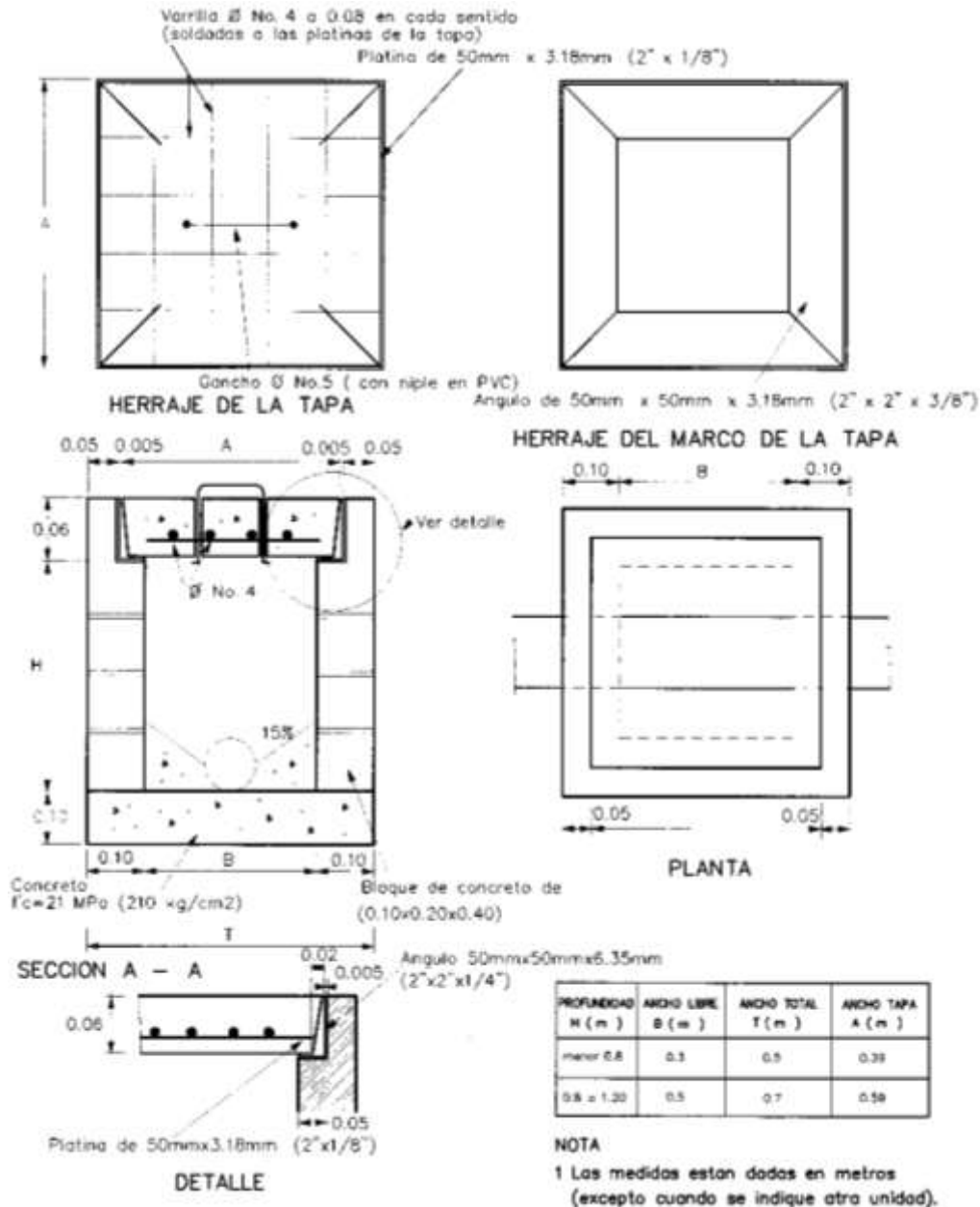
Esquema 60. Caja de empalme para la domiciliaria en Andén o zona verde
