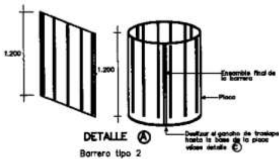
BARRERA CIRCULAR PARA CONTROL RADICULAR
