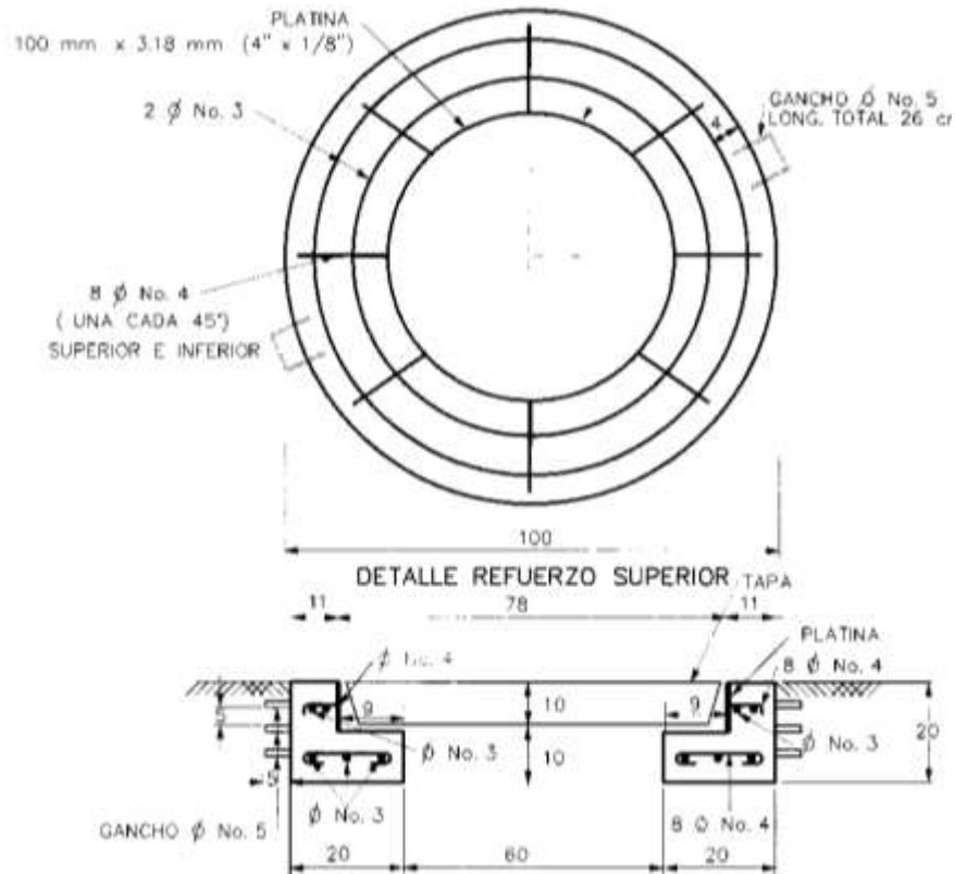
Esquema 52. Anillo para tapa de concreto
