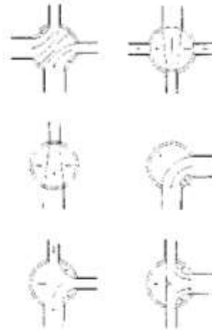
CASOS TÍPICOS DE CAÑUELAS
