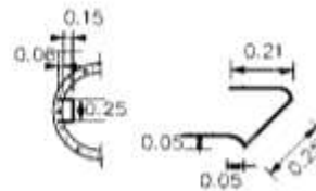
DETALLE PELDAÑO
