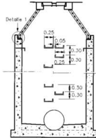
SECCION A-A DETALLE ③ COLOCACIÓN PELDAÑOS
