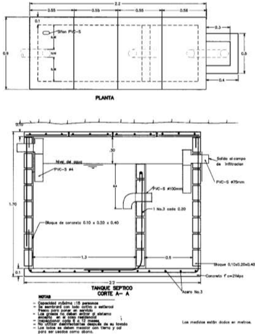
Esquema 1. Tanque Séptico
