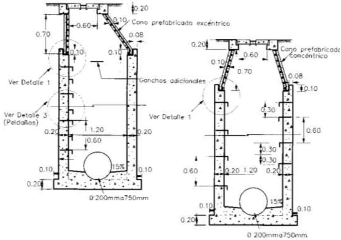
CÁMARA EXCÉNTRICA
