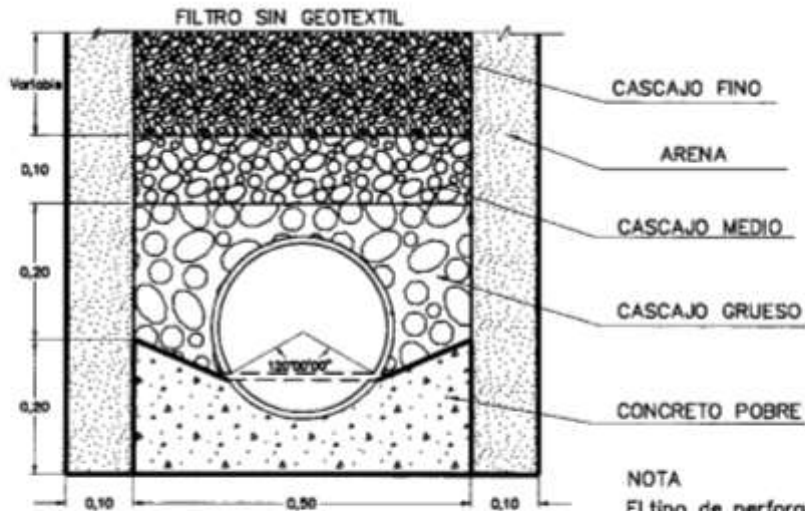
DETALLE DRENES Y FILTROS
