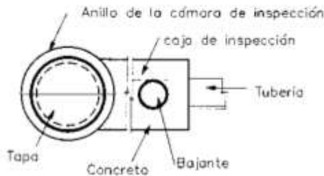
SECCION A - A
