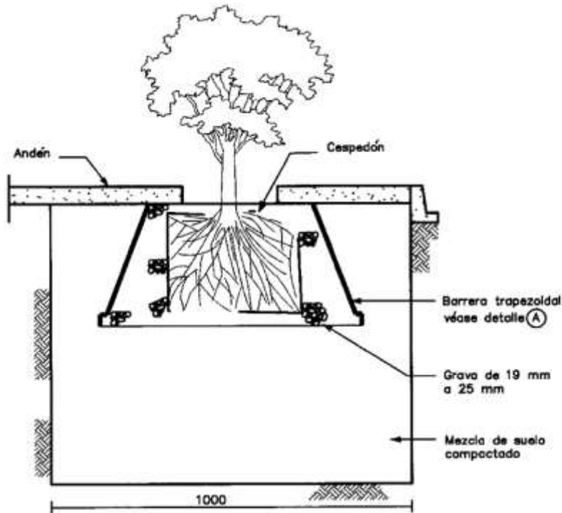
BARRERA TRAPEZOIDAL PARA CONTROL RADICULAR
