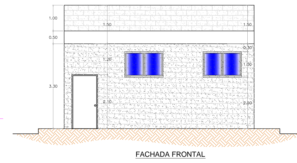
CASETA DE CLORACIÓN
