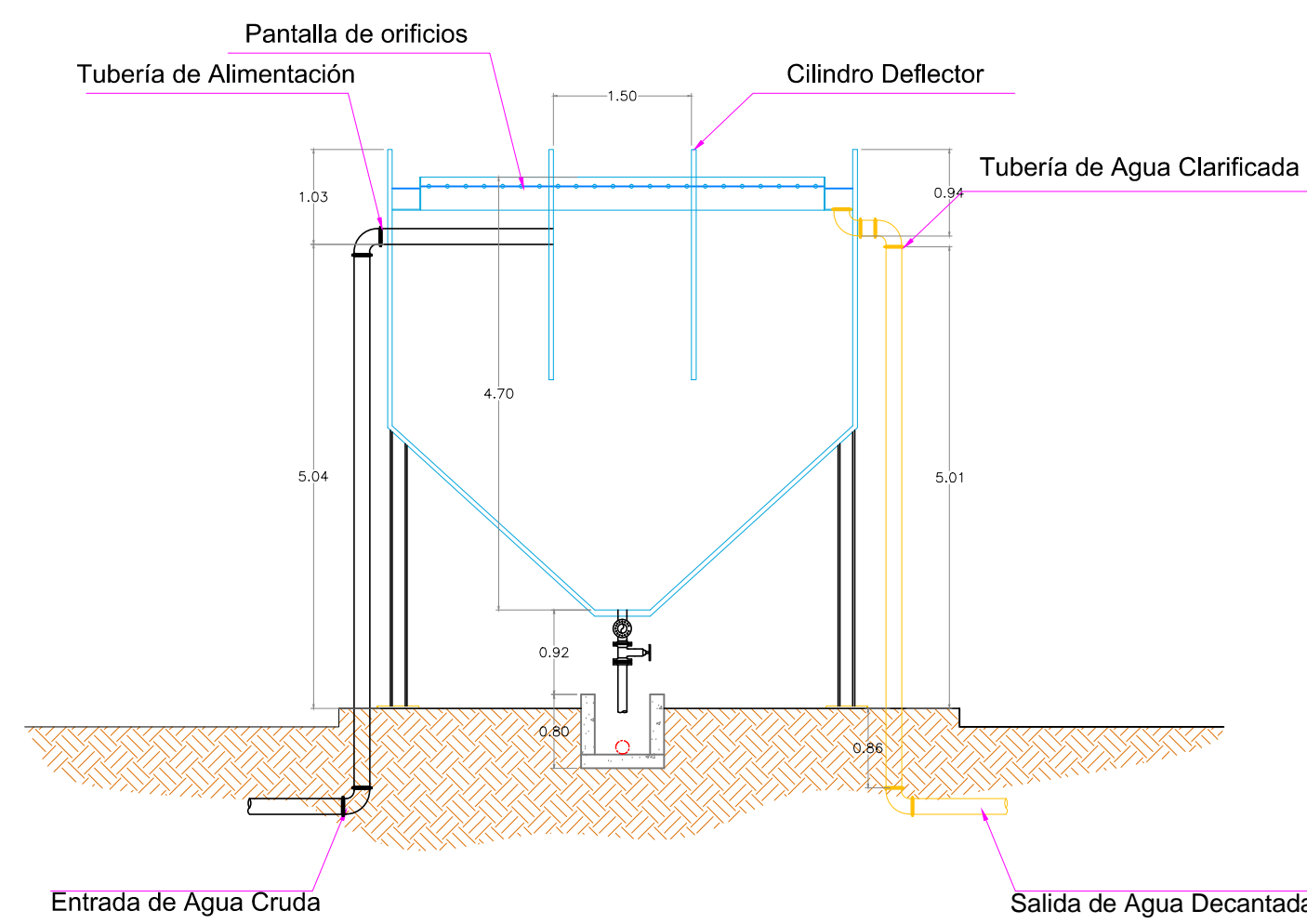
DETALLES DE LOS ESPESADORES
