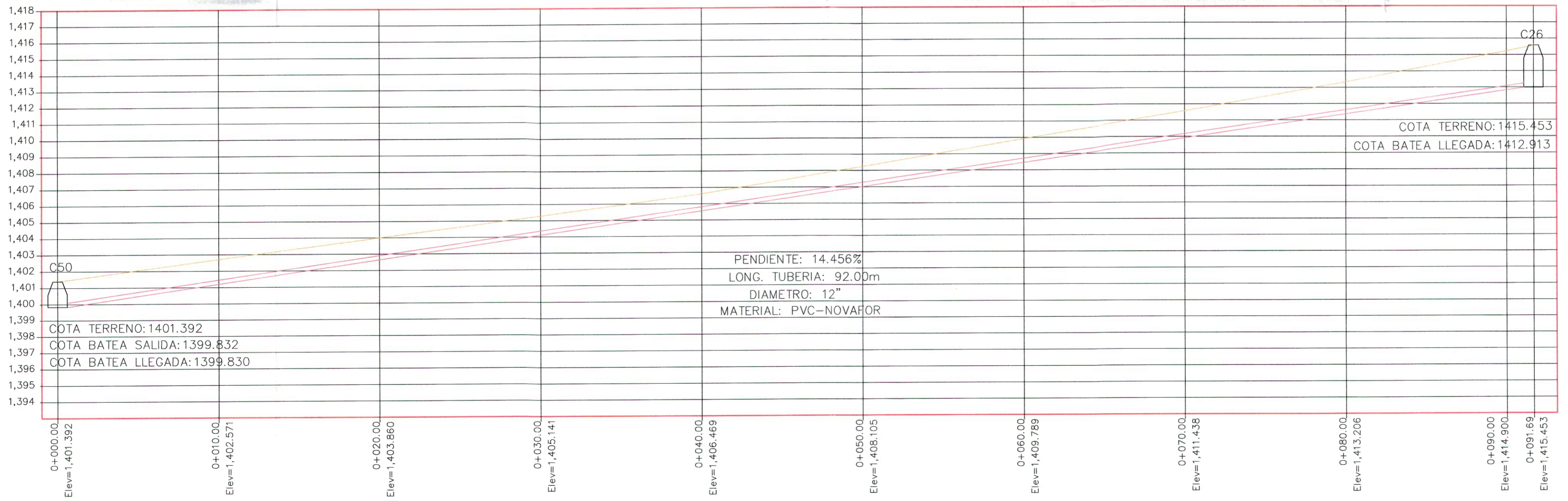
PERFIL CALLE 46-47 CARRERA 51 ESCALA HORIZONTAL 1 : 1000 ESCALA VERTICAL 1 : 1000
