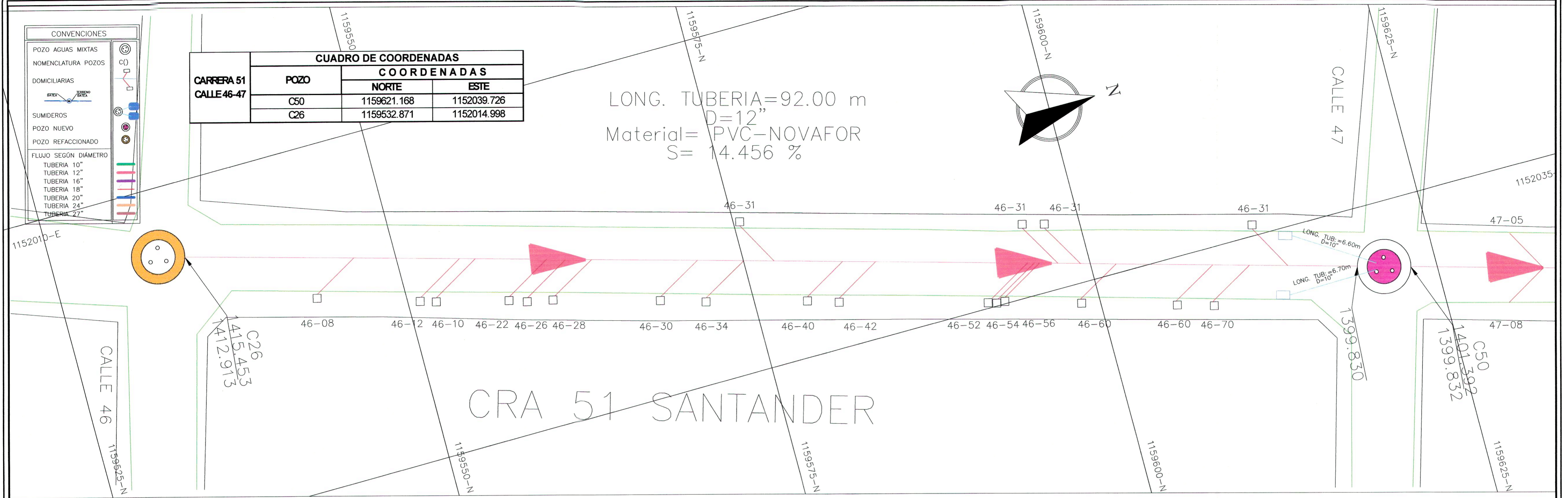
TRAMO DISEÑO CARRERA 51 CALLE 46-47
