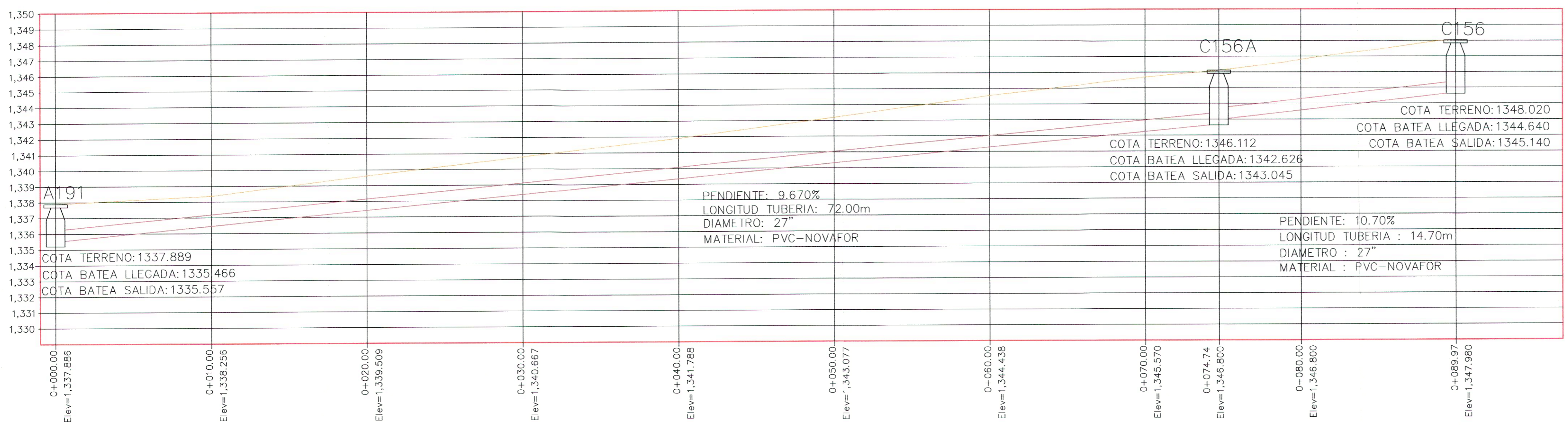
PERFIL CARRERA 52 CALLE 51-52 ESCALA HORIZONTAL 1 : 1000 ESCALA VERTICAL 1 : 1000
