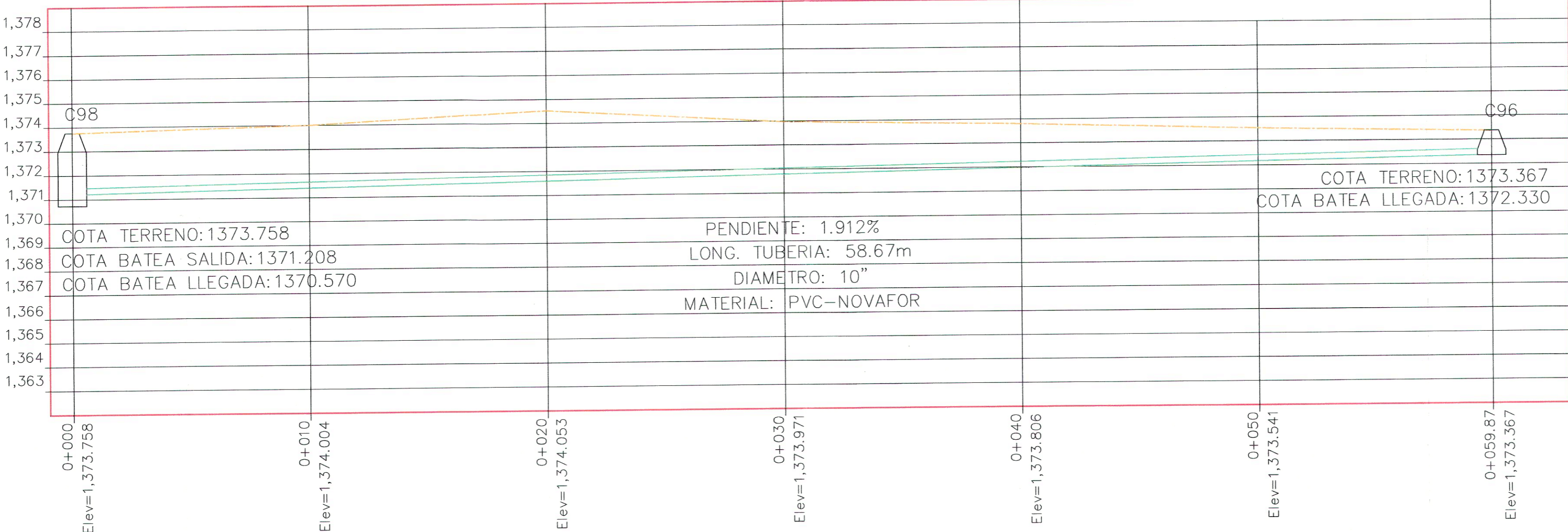
PERFIL CALLE 49 CARRERA 53-52 ESCALA HORIZONTAL 1 : 1000 ESCALA VERTICAL 1 : 1000
