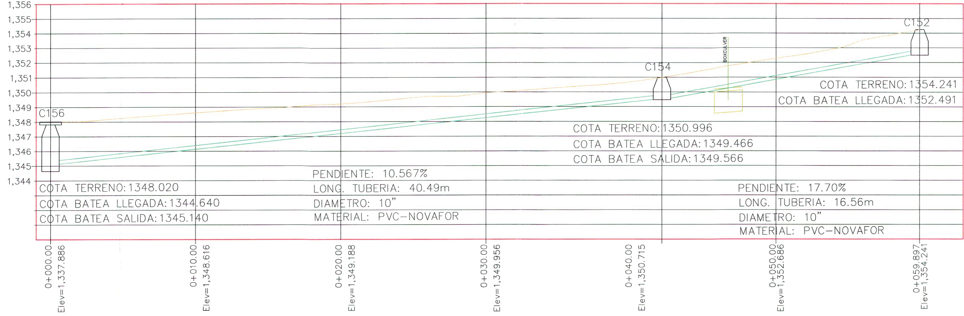
PERFIL CALLE 51 CARRERA 52-53 ESCALA HORIZONTAL 1 : 1000 ESCALA VERTICAL 1 : 1000
