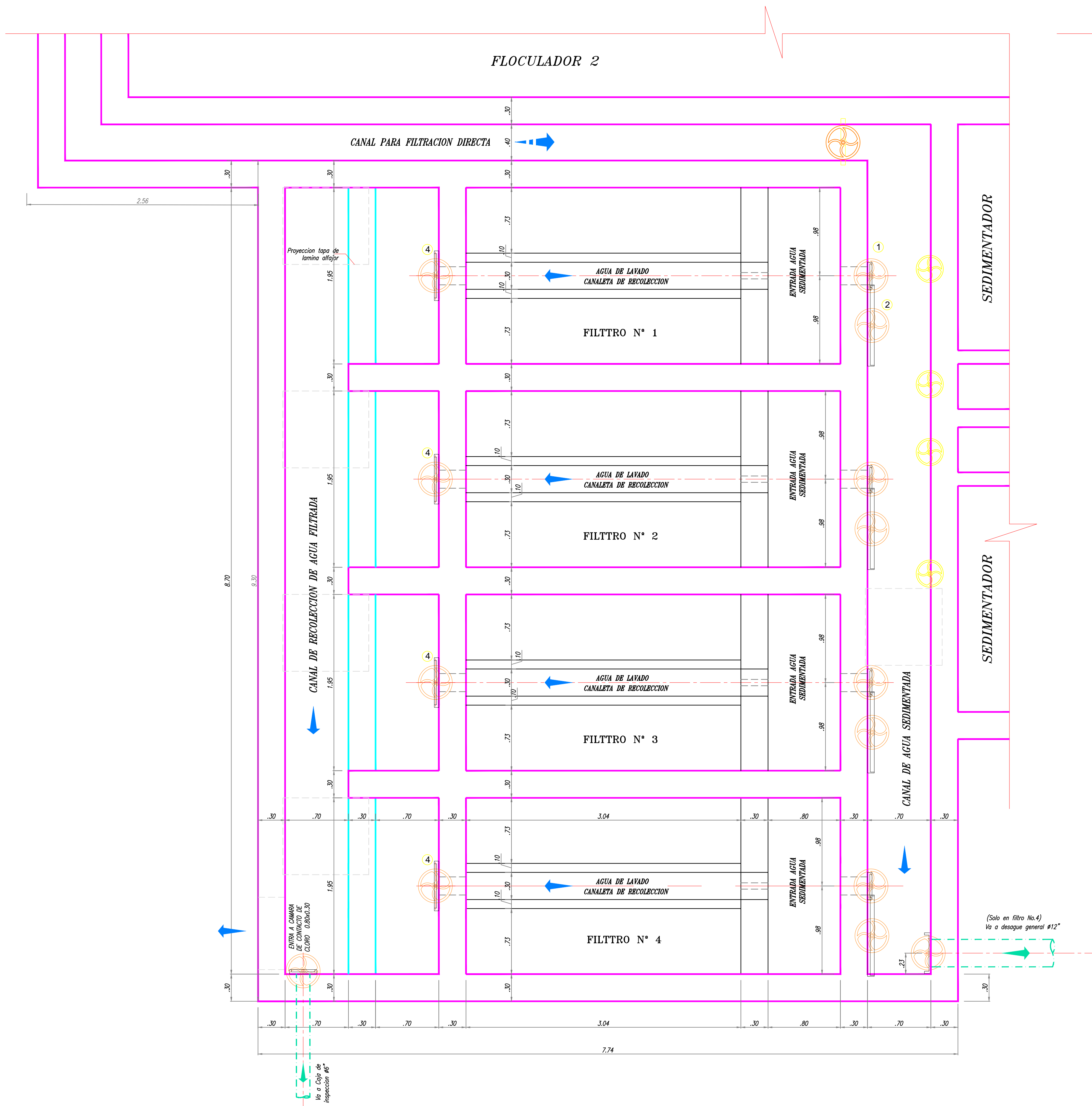
PLANTA BATERIA DE FILTROS
