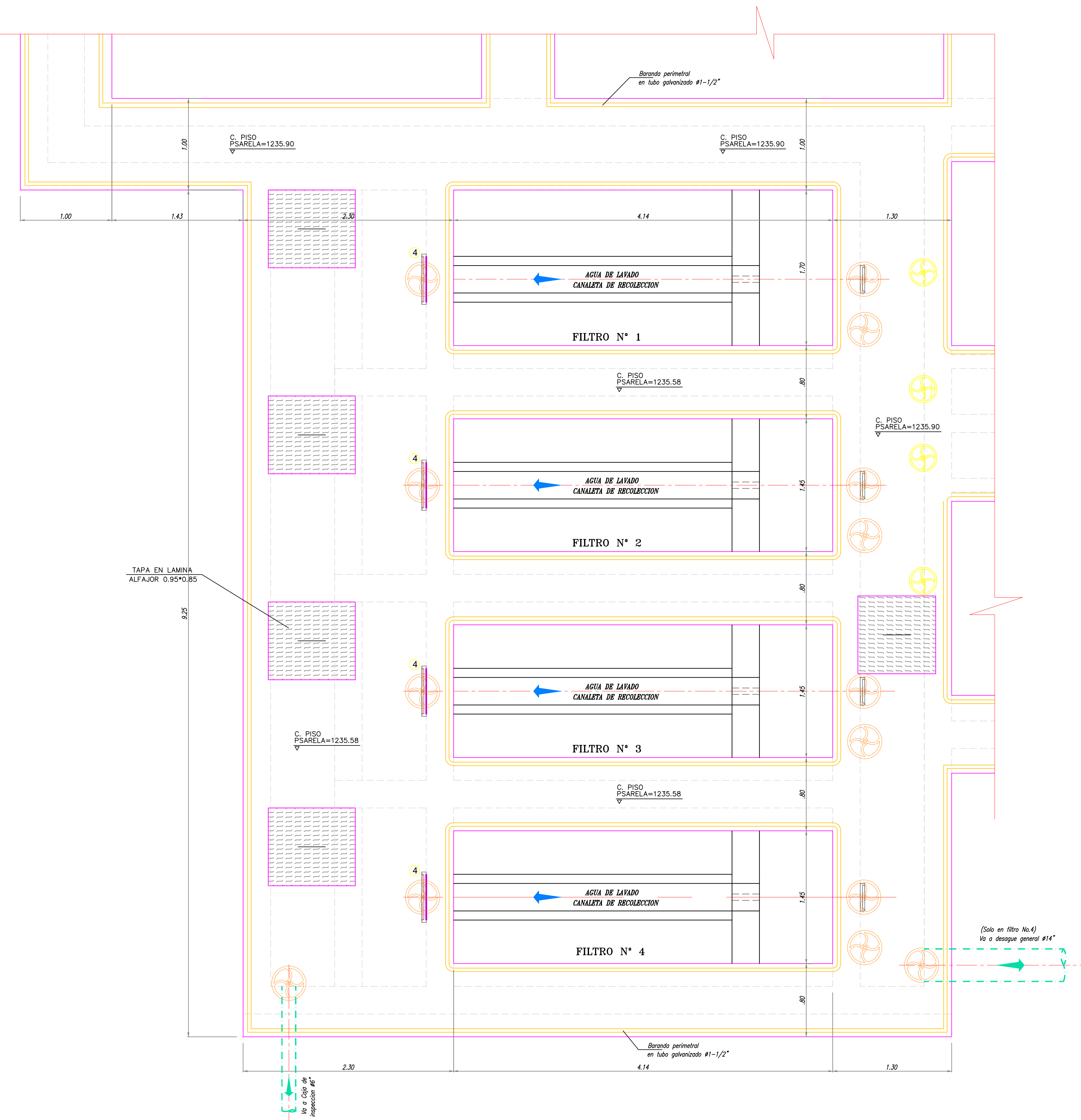
PLANTA PASARELA FILTROS
