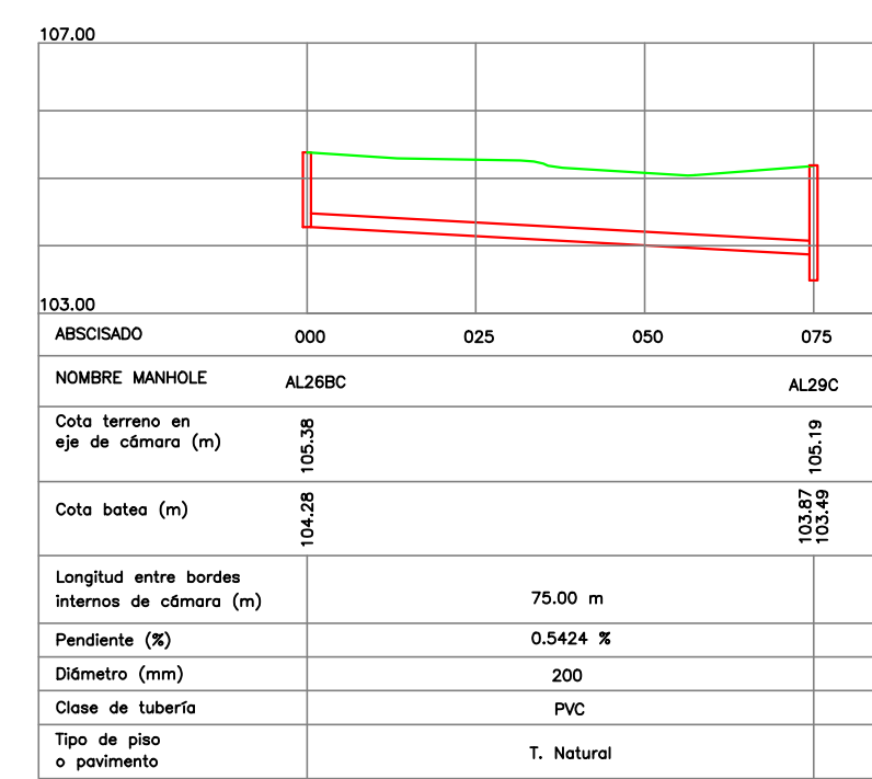
PERFIL MANHOLES AL28C - AL29C
