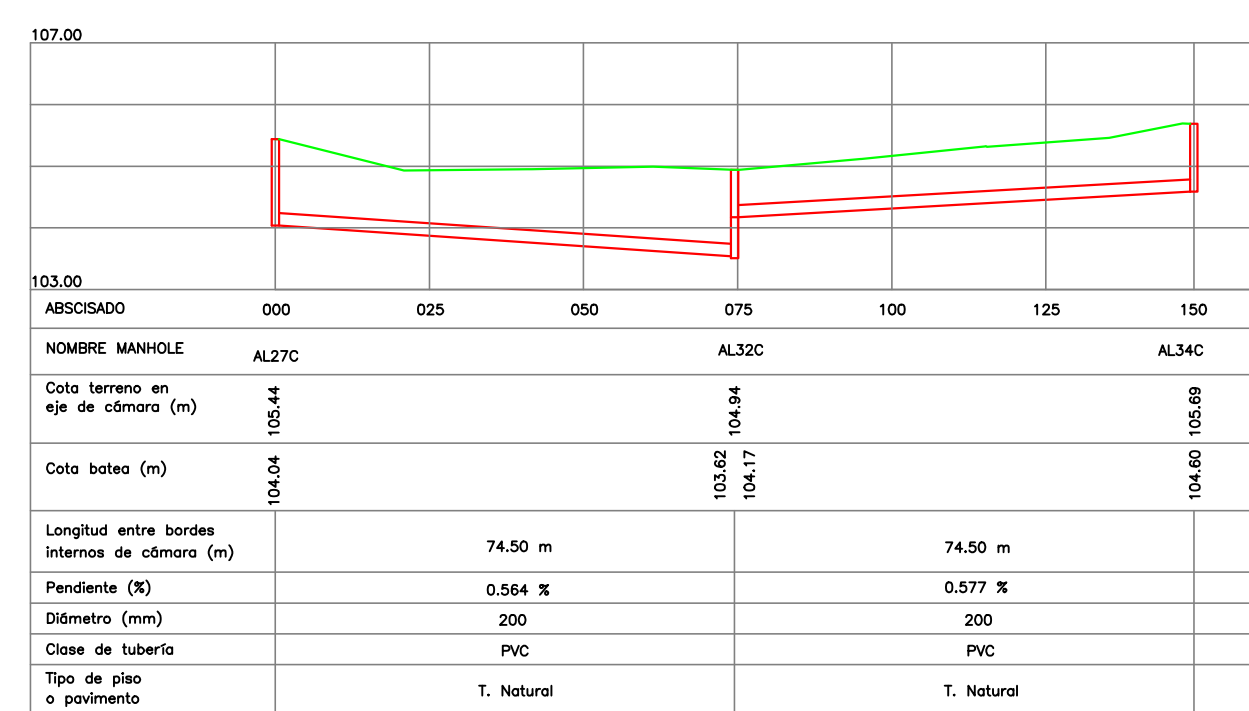
PERFIL MANHOLES AL27C - AL34C
