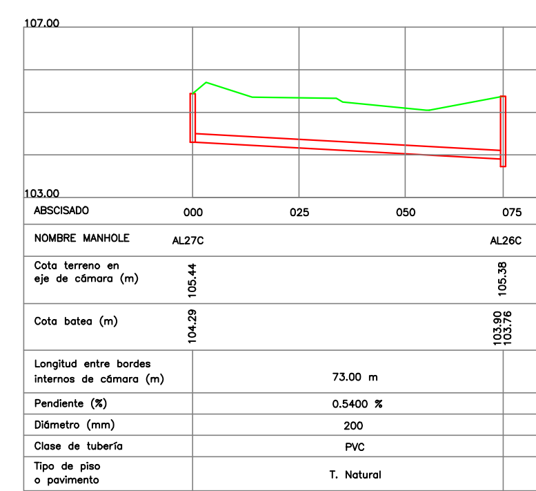
PERFIL MANHOLES AL27C - AL28C
