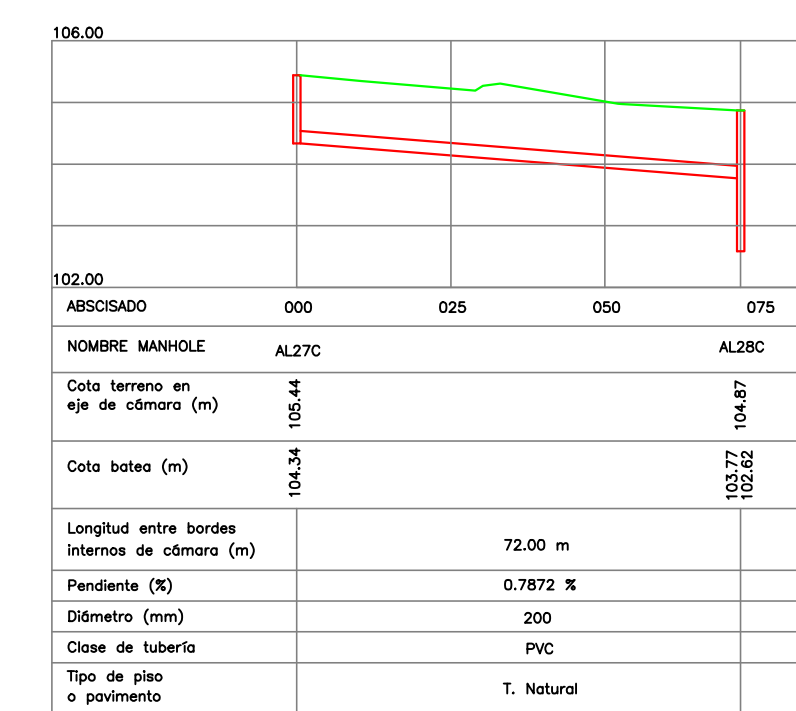
PERFIL MANHOLES AL27C - AL28C
