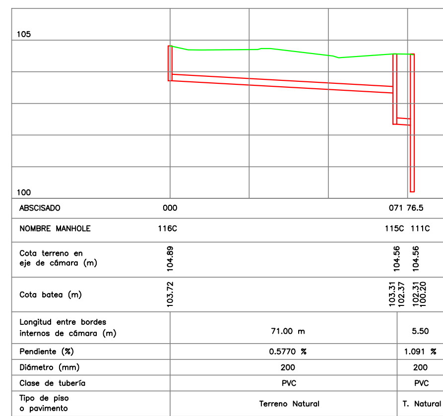
PERFIL MANHOLES 116C - 111C
