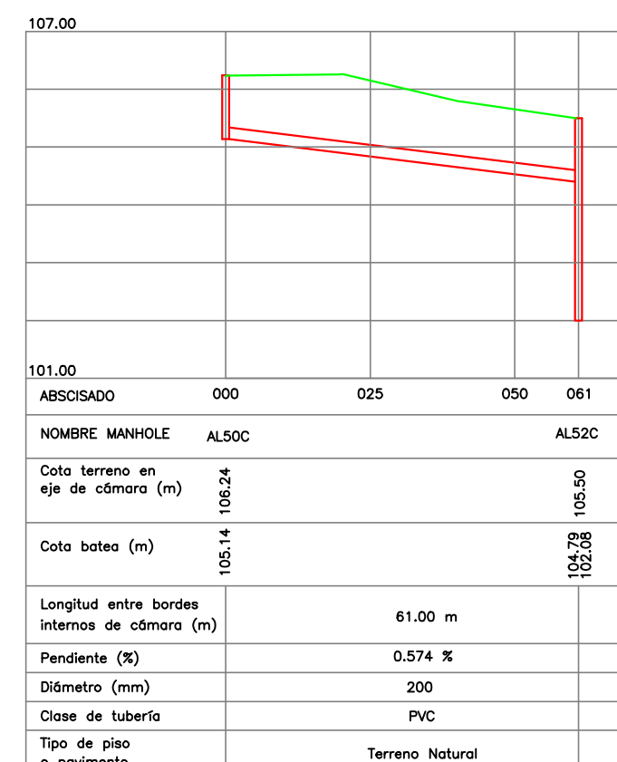
PERFIL MANHOLES AL50C - AL52C
