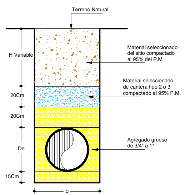
CIMENTACIÓN TÍPICA TUBERÍA CON PRESENCIA DE NIVEL FREÁTICO PROFUNDIDAD MAYOR A 1,6 M (TEÓRICO)
