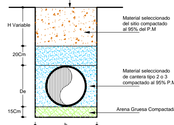
CIMENTACIÓN TÍPICA TUBERÍA SIN PRESENCIA DE NIVEL FREÁTICO PROFUNDIDAD MENOR A 1,6 M (TEÓRICO)
