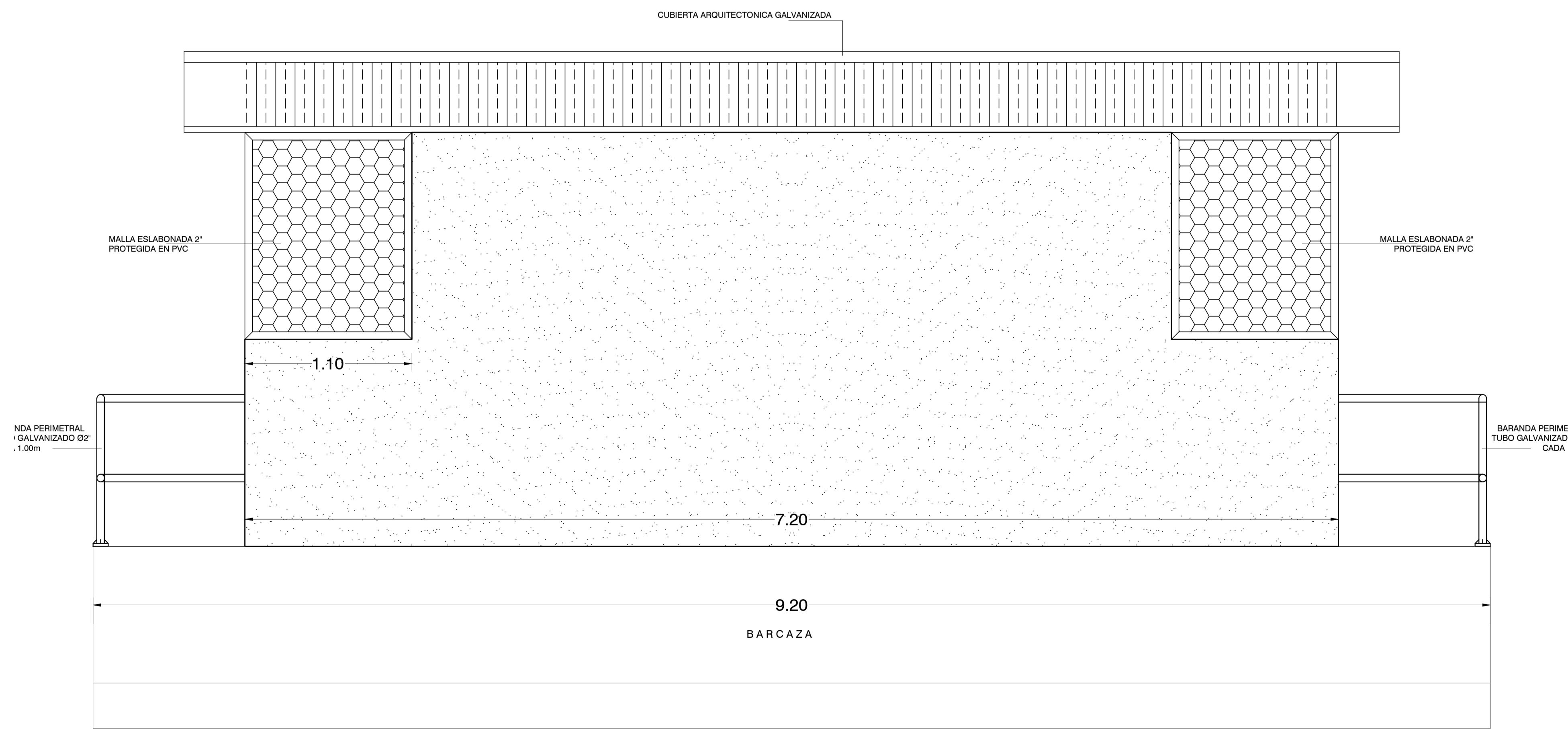
FACHADA POSTERIOR ESC: 1:20
