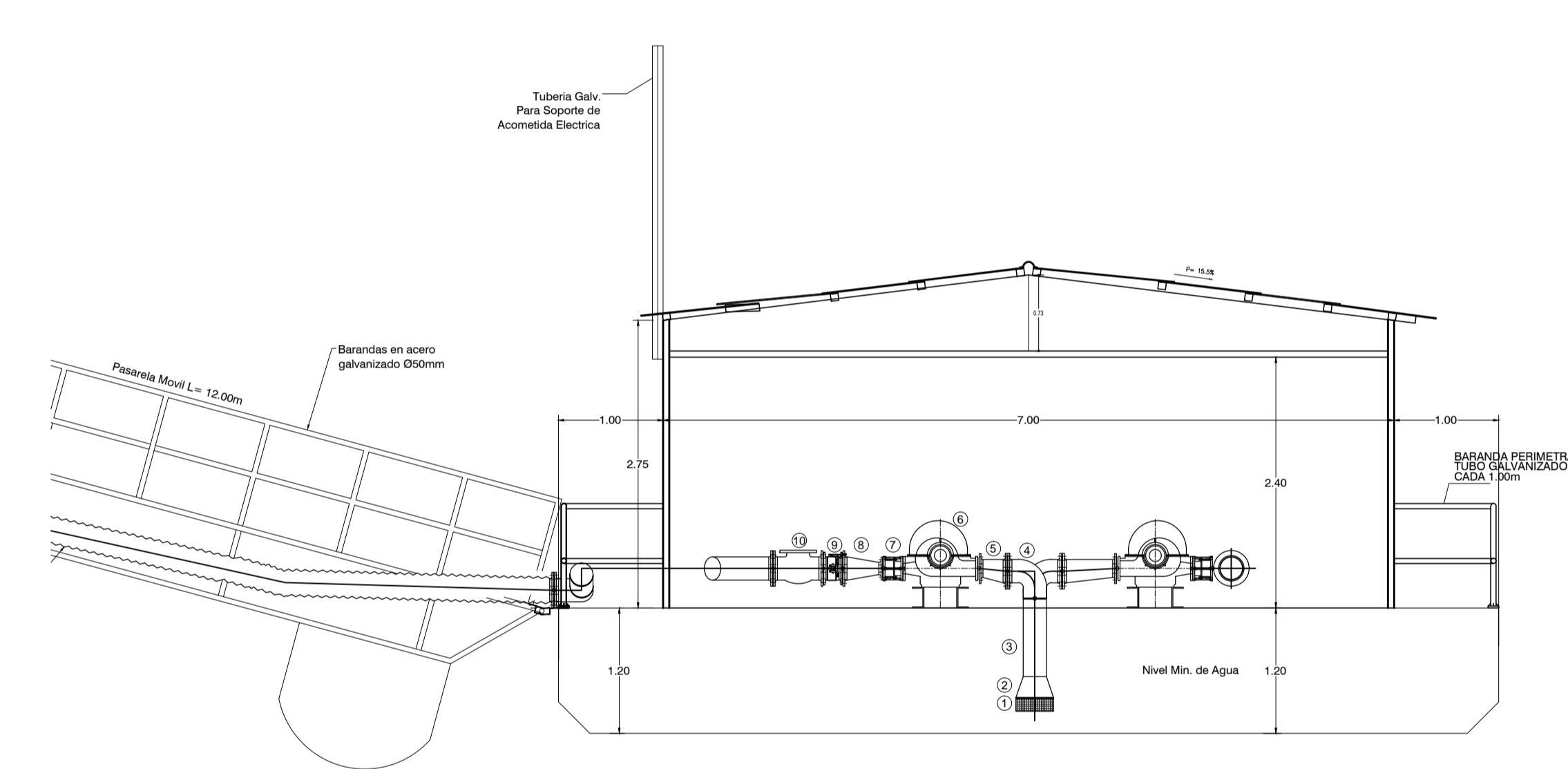
SECCION BARCAZA ESC: 1/50
