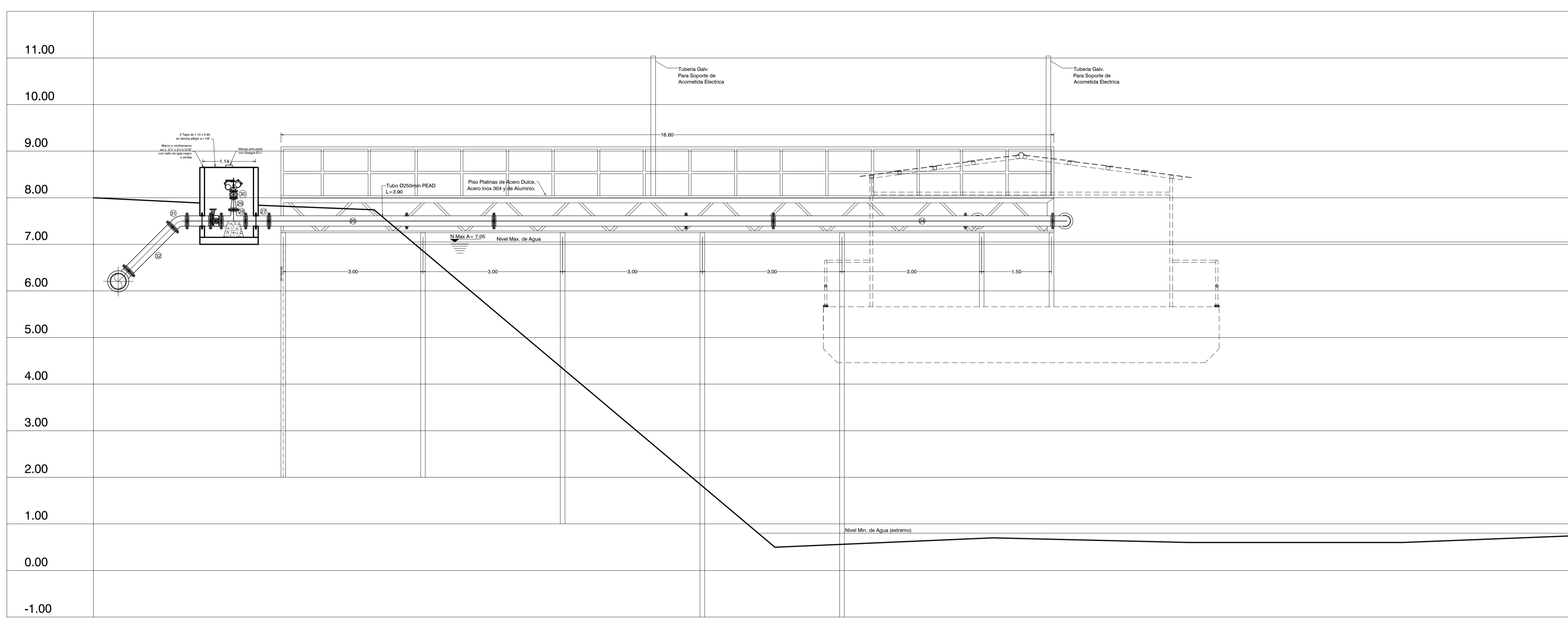
SECCION A - A ESC: 1:50
