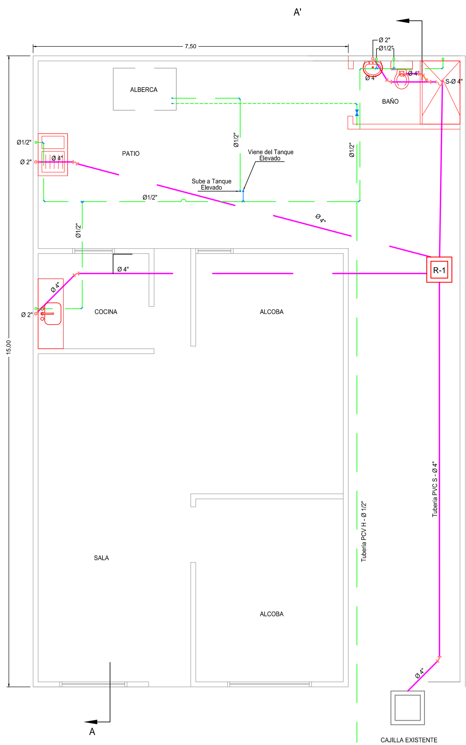
J. INTERVENCIÓN 5 APARATOS BAÑO PATIO
