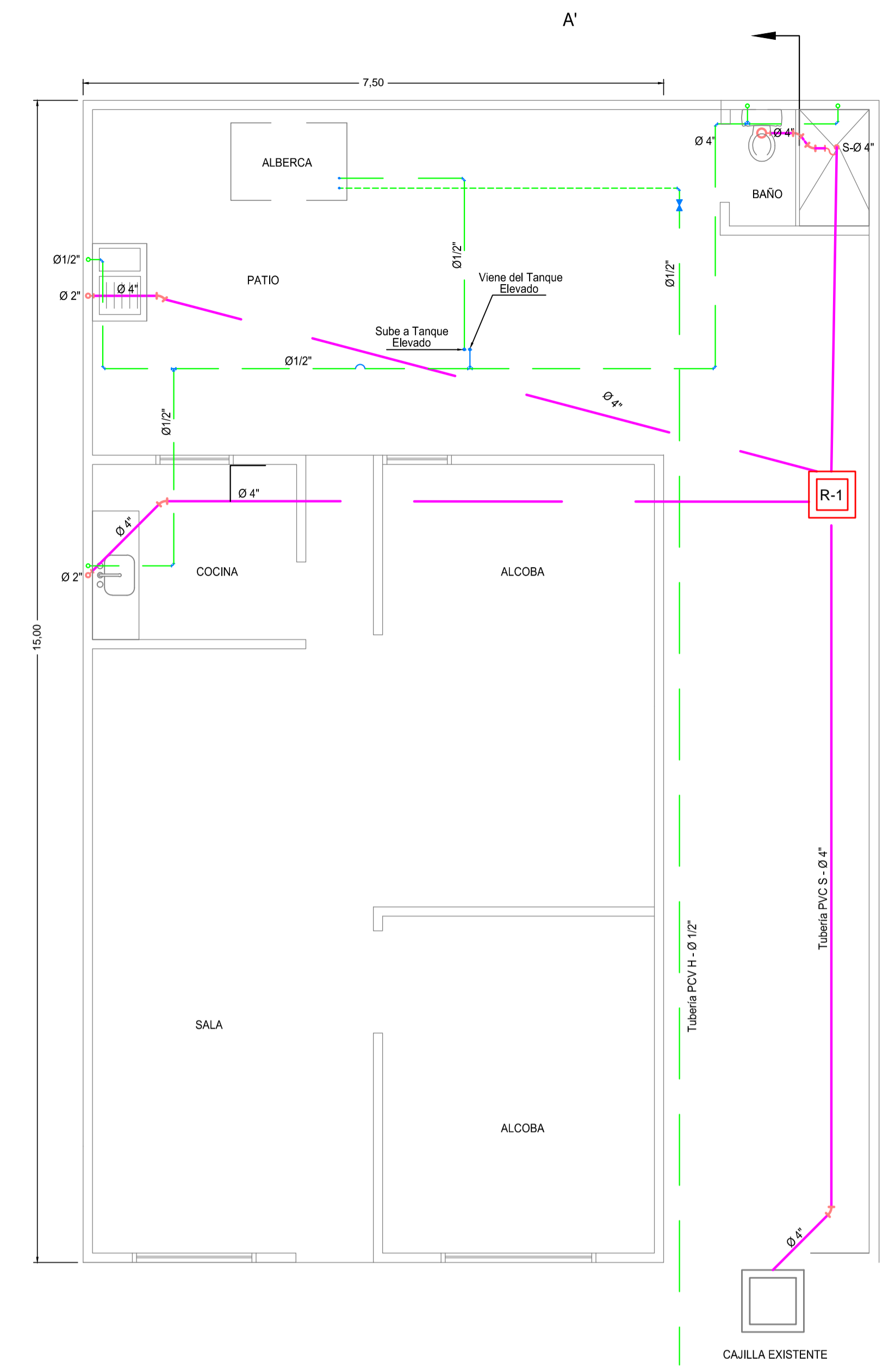
A. INTERVENCIÓN REDES INTERNAS
