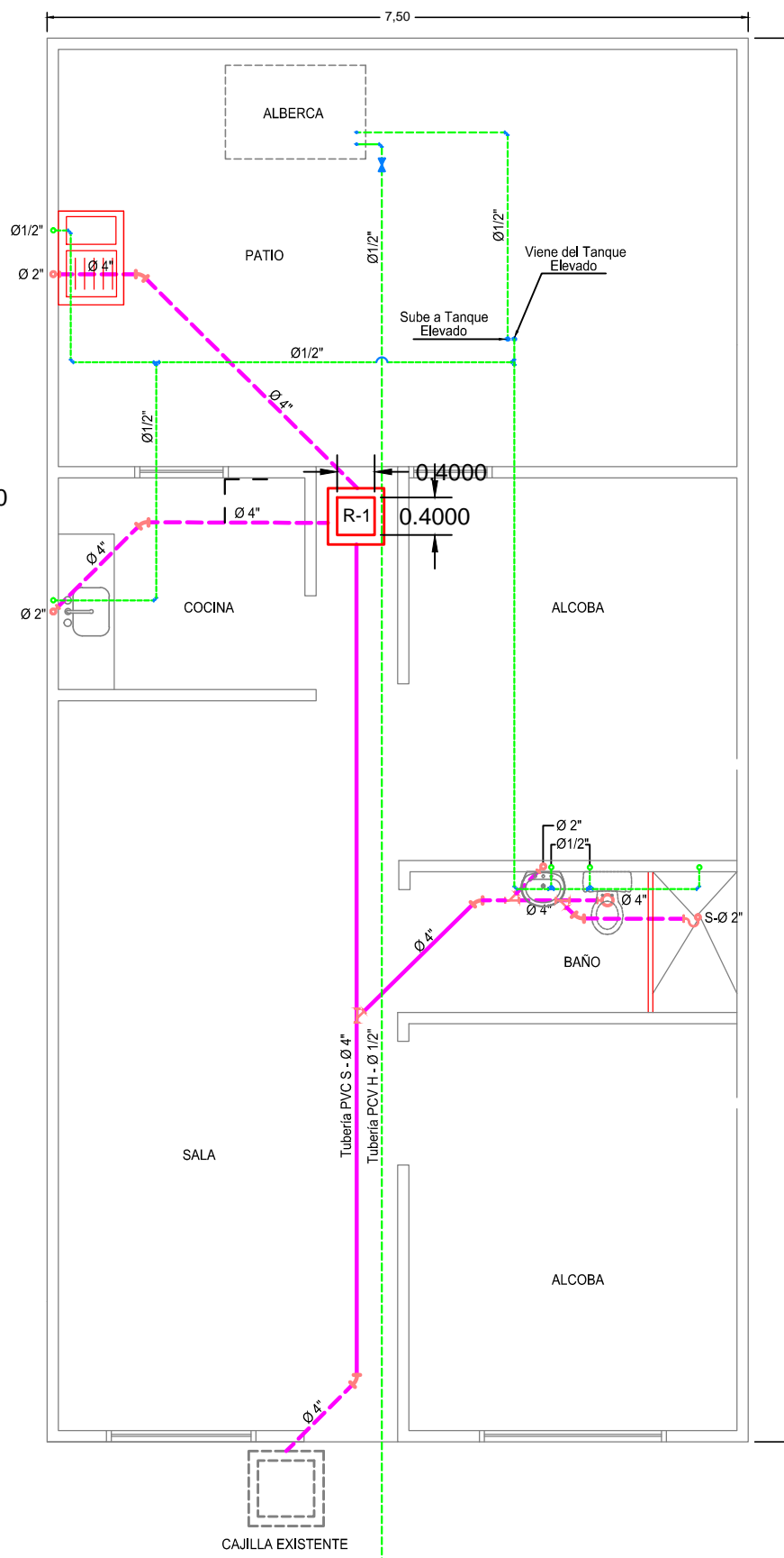
C. INTERVENCIÓN 1 APARATO BAÑO INTERNO
