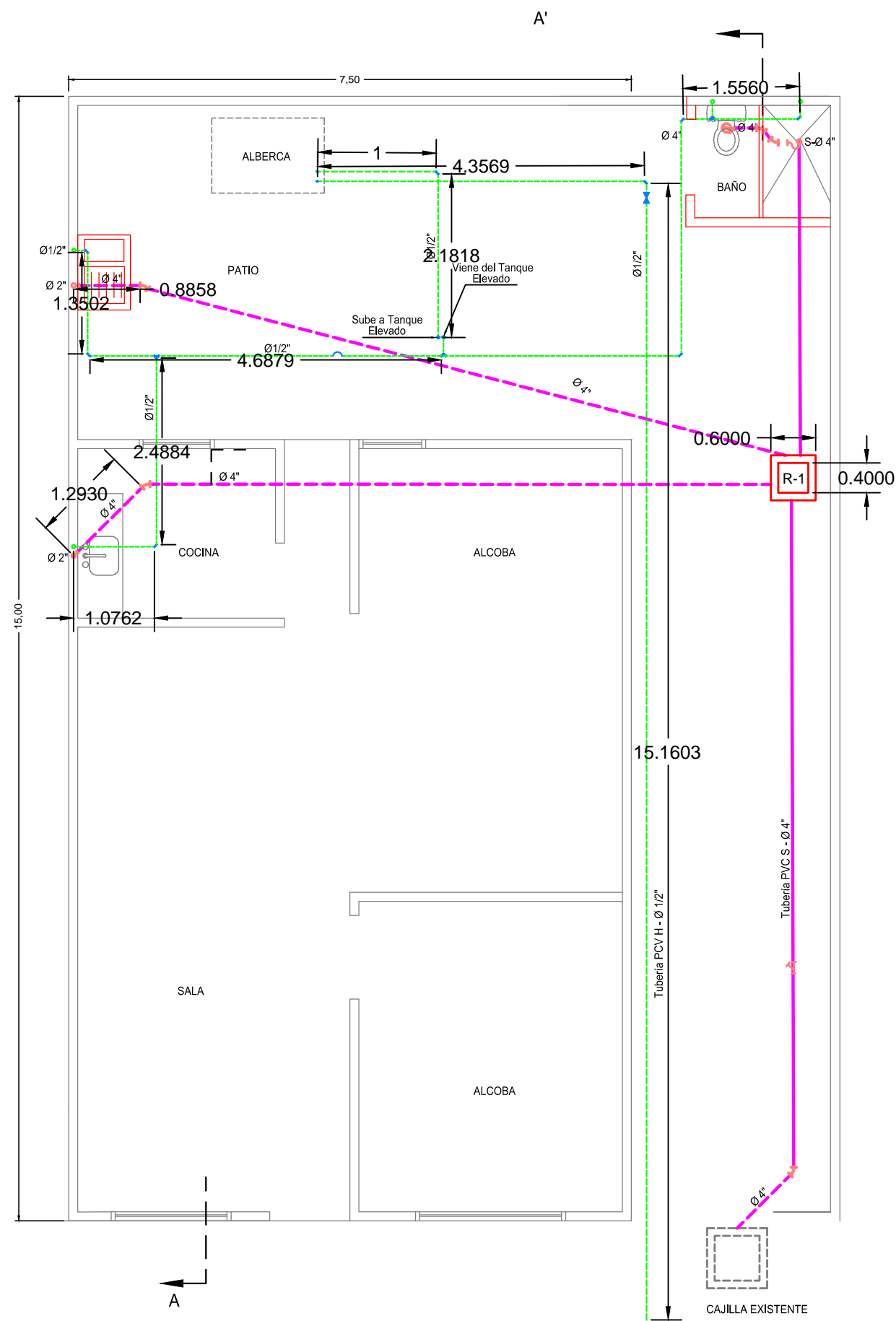
B. INTERVENCIÓN 1 APARATO BAÑO PATIO
