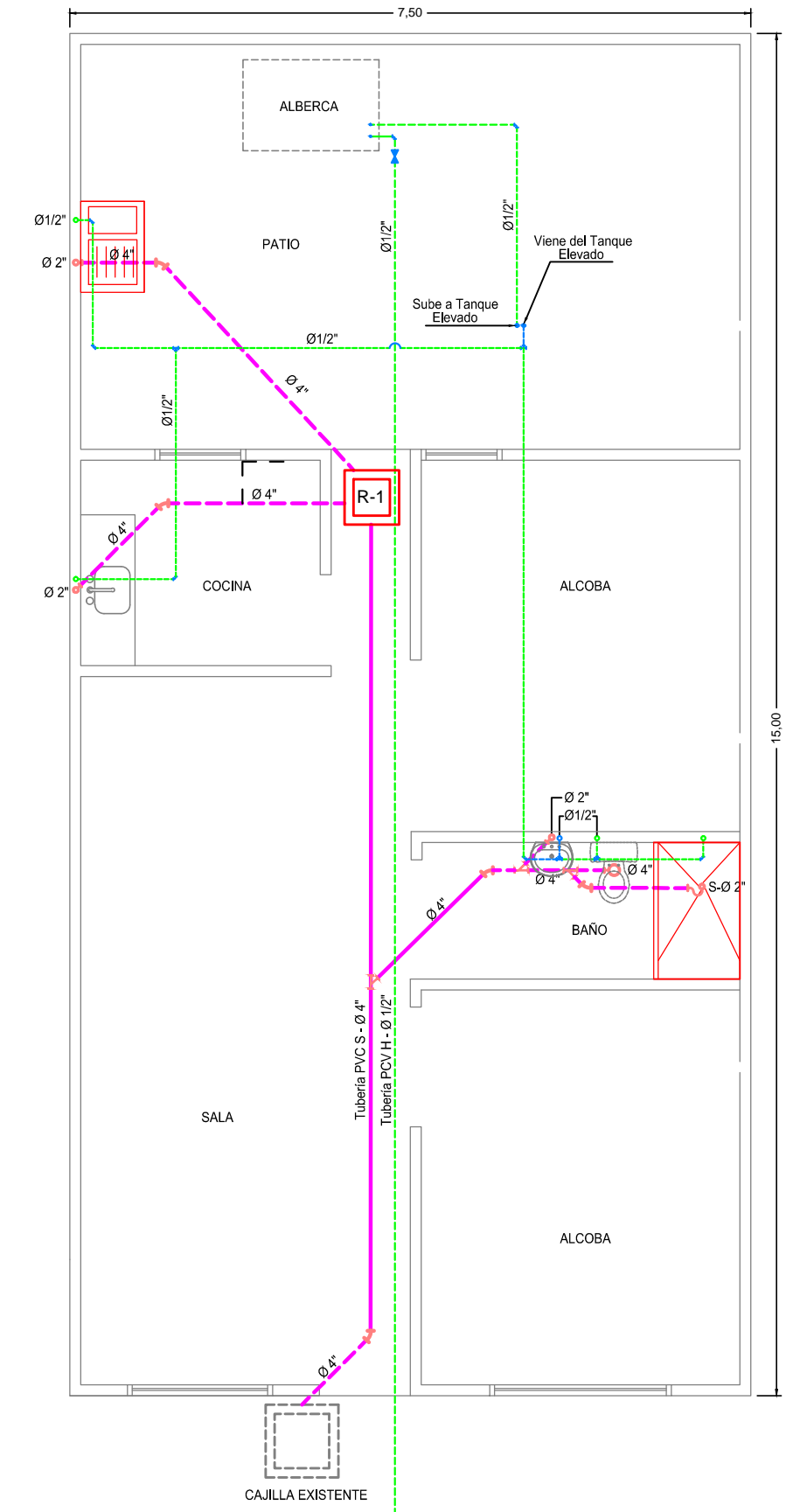
E. INTERVENCIÓN 2 APARATO BAÑO INTERNO
