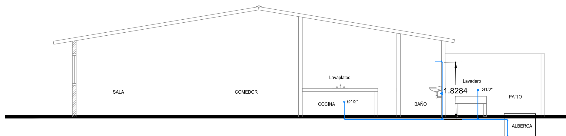
SECCIÓN CORTE A - A' VIVIENDA ESCALA 1:50
