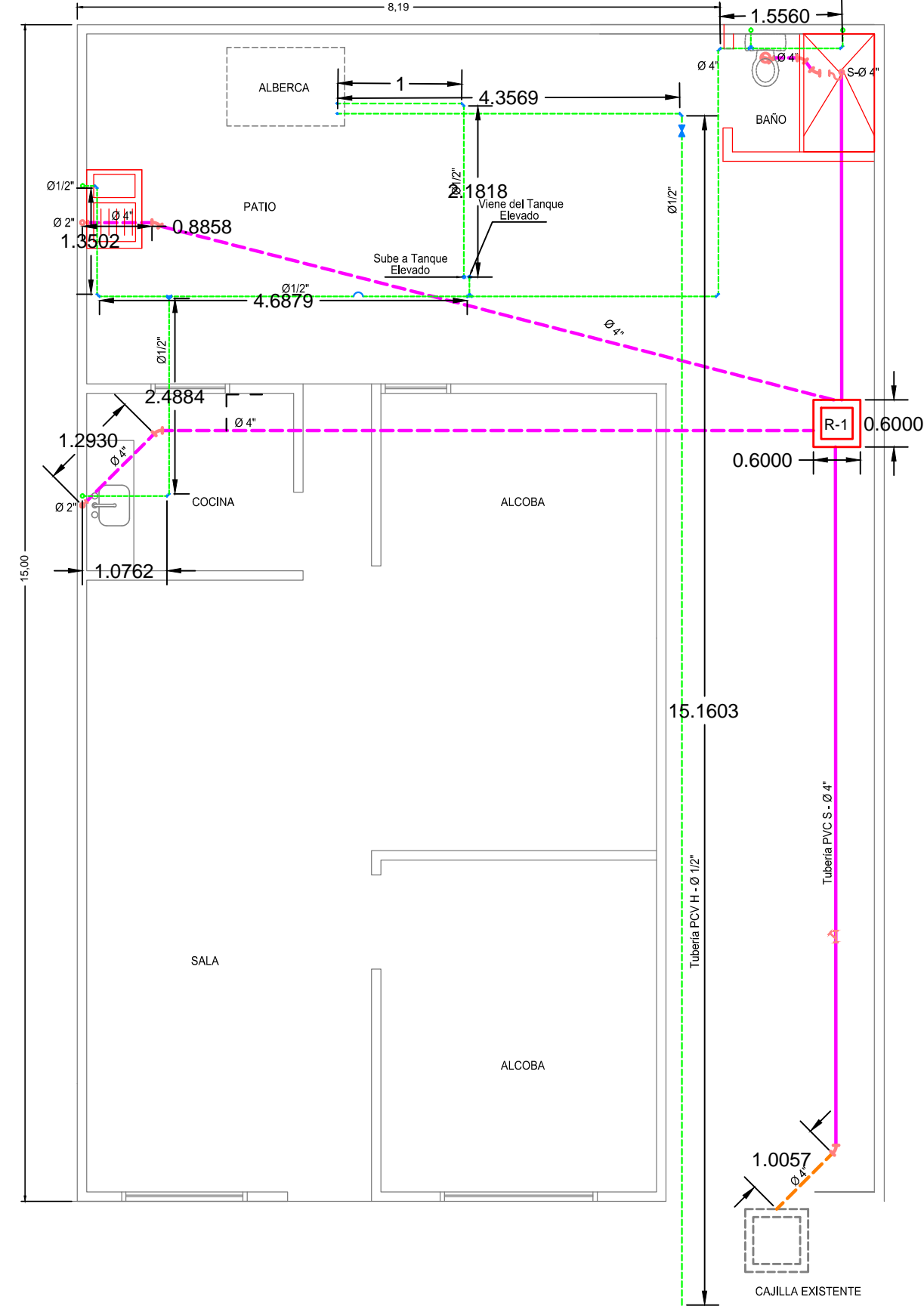
D. INTERVENCIÓN 2 APARATO BAÑO PATIO
