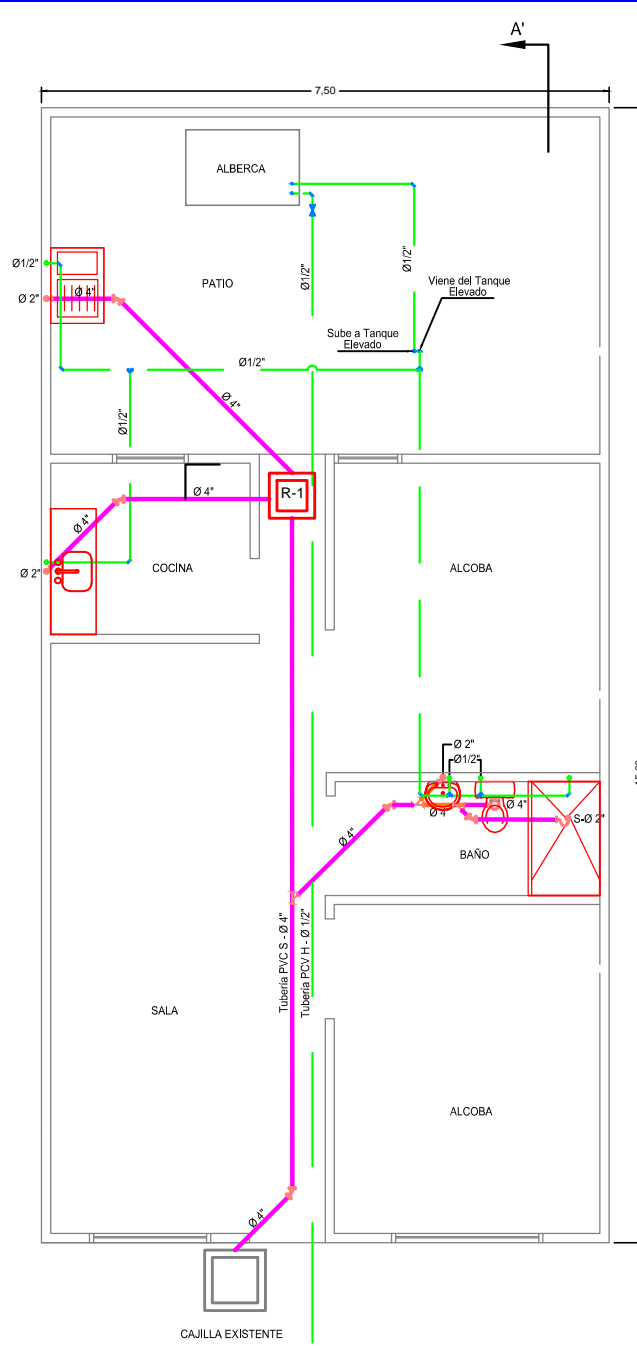
K. INTERVENCIÓN 5 APARATOS BAÑO INTERNO
