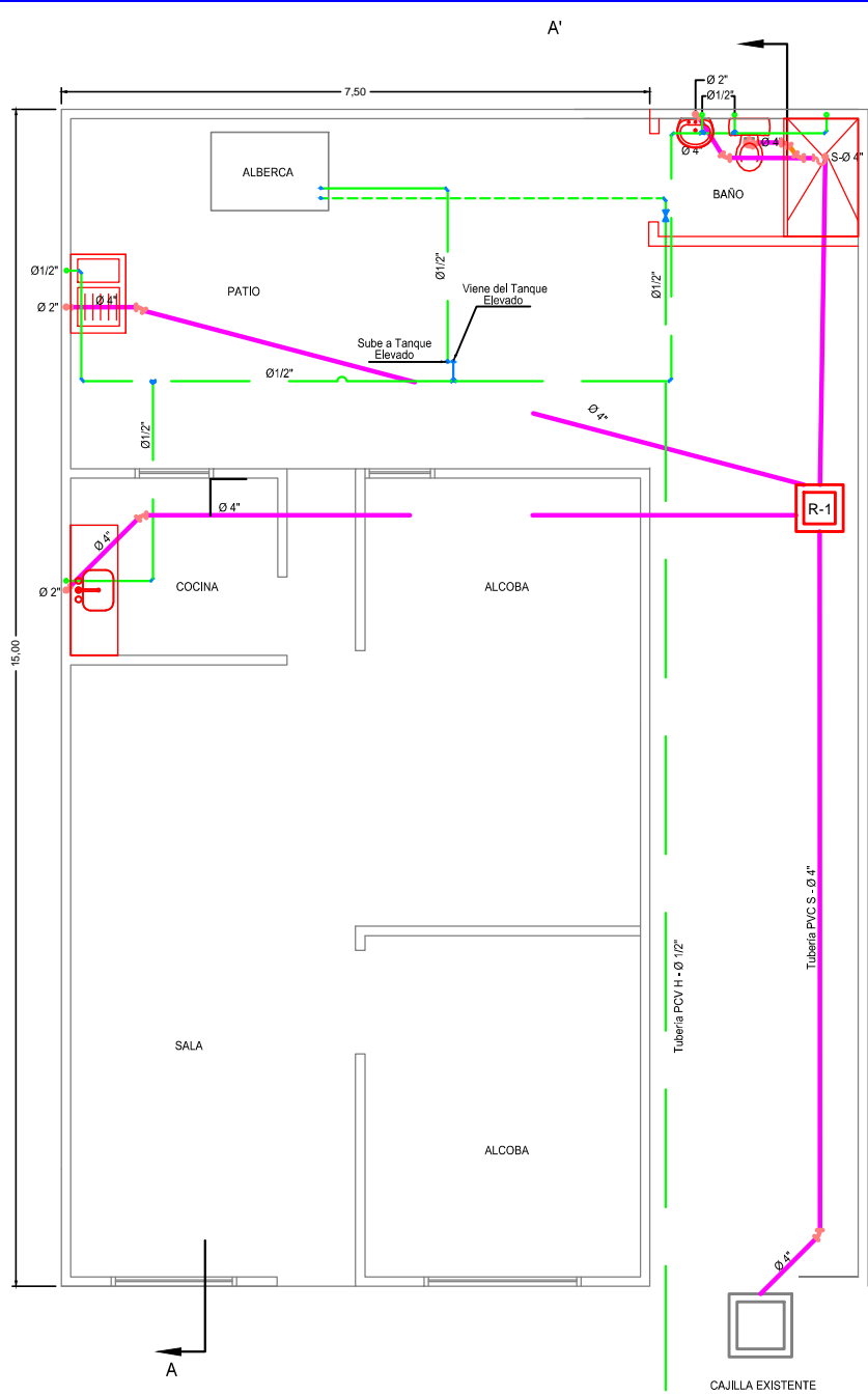
J. INTERVENCIÓN 5 APARATOS BAÑO PATIO
