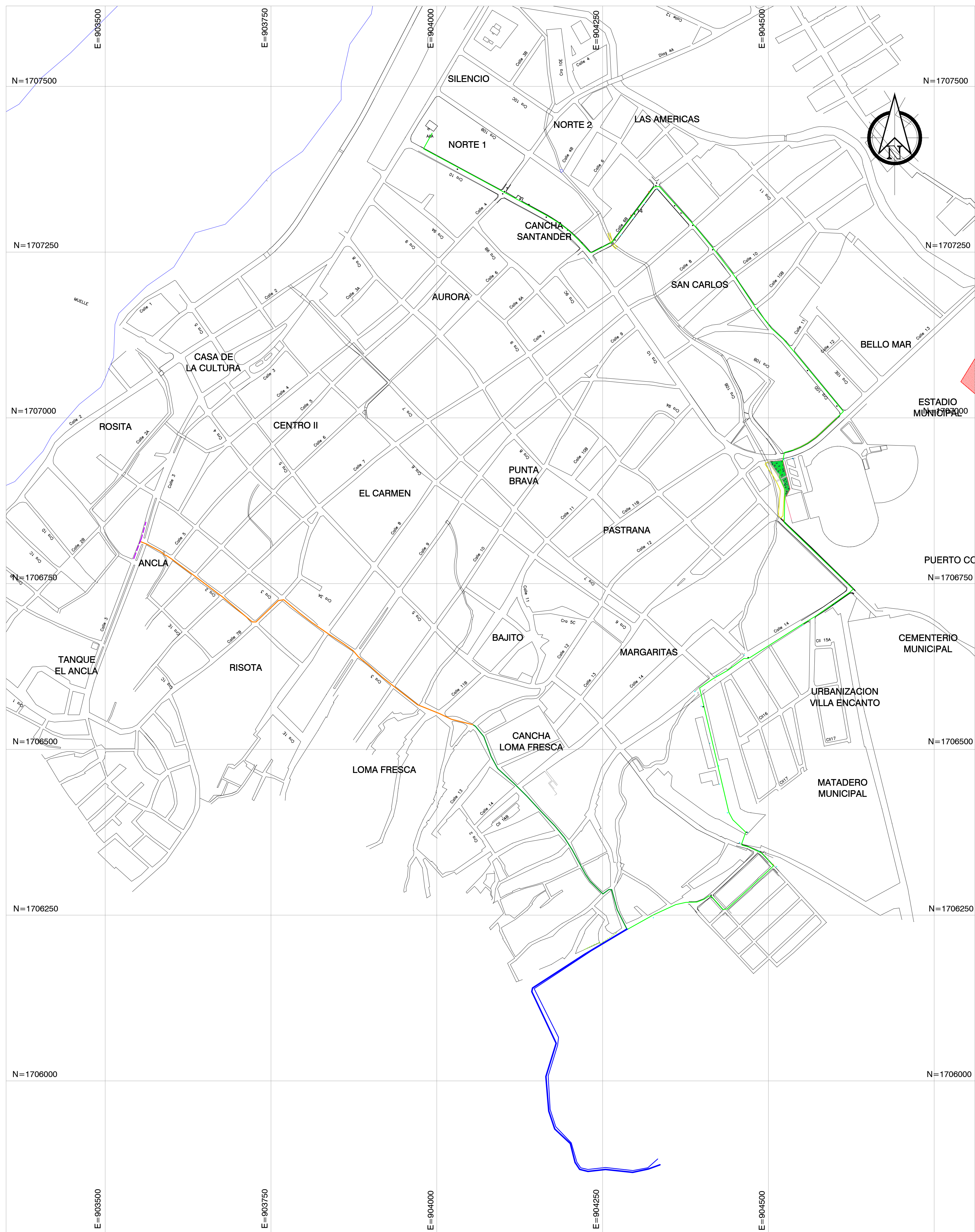
LOCALIZACION DE TUBERIAS DE IMPULSION Y CONDUCCION MUNICIPIO DE PUERTO COLOMBIA ESC: _____ S/E
