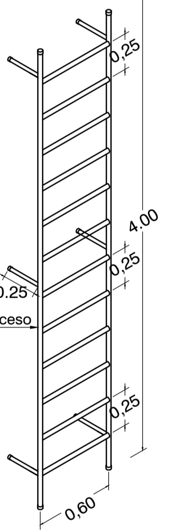
DETALLE ESCALERA DE ACCESO
