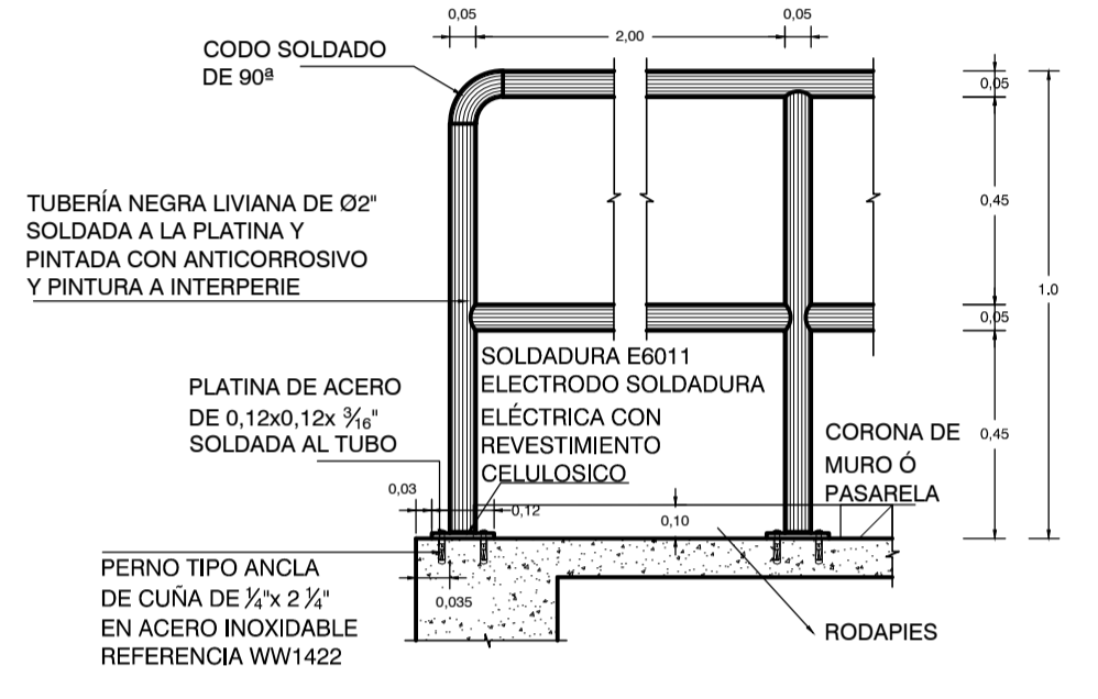
FIJACION PASAMANOS
