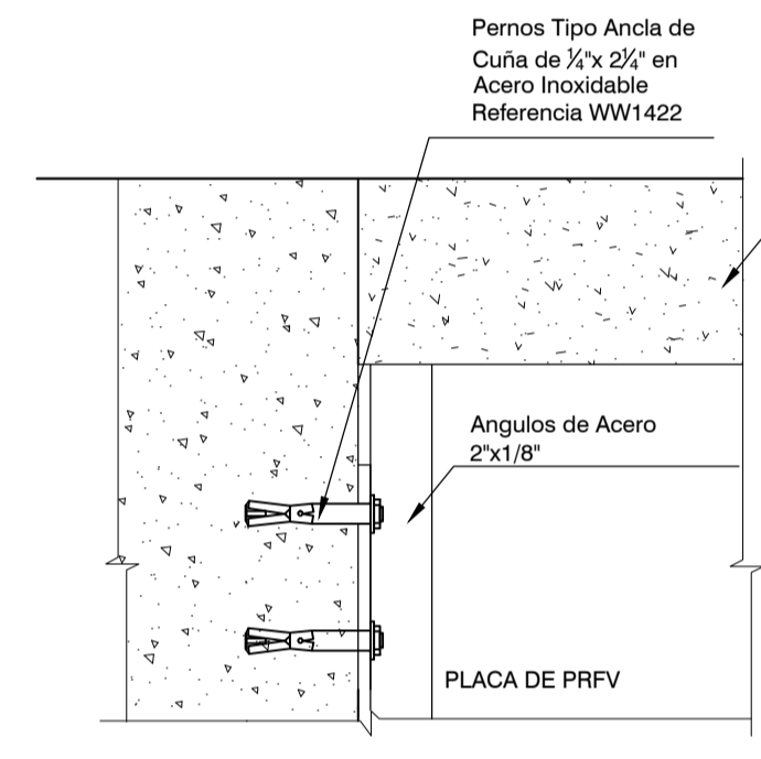
VISTA FRONTAL ESC. 5/E
