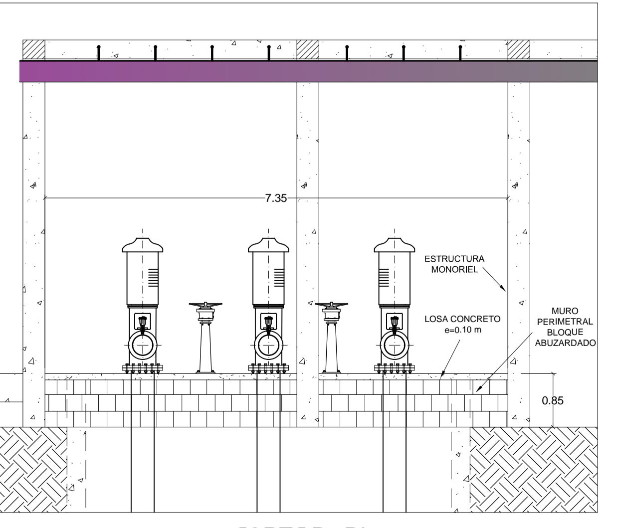
CORTE D - D' ESC. 5/E
