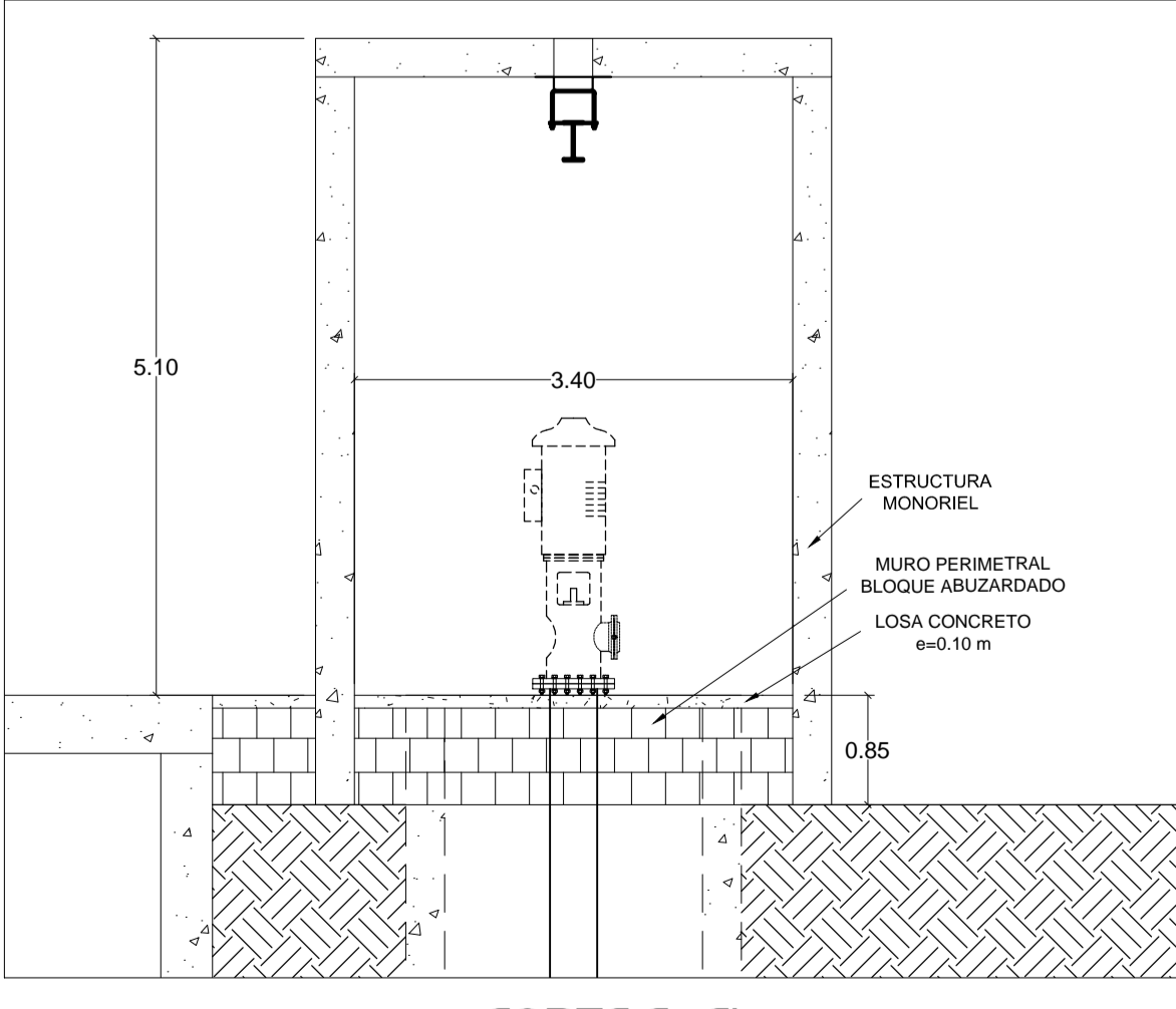
CORTE C - C' ESC. 5/E
