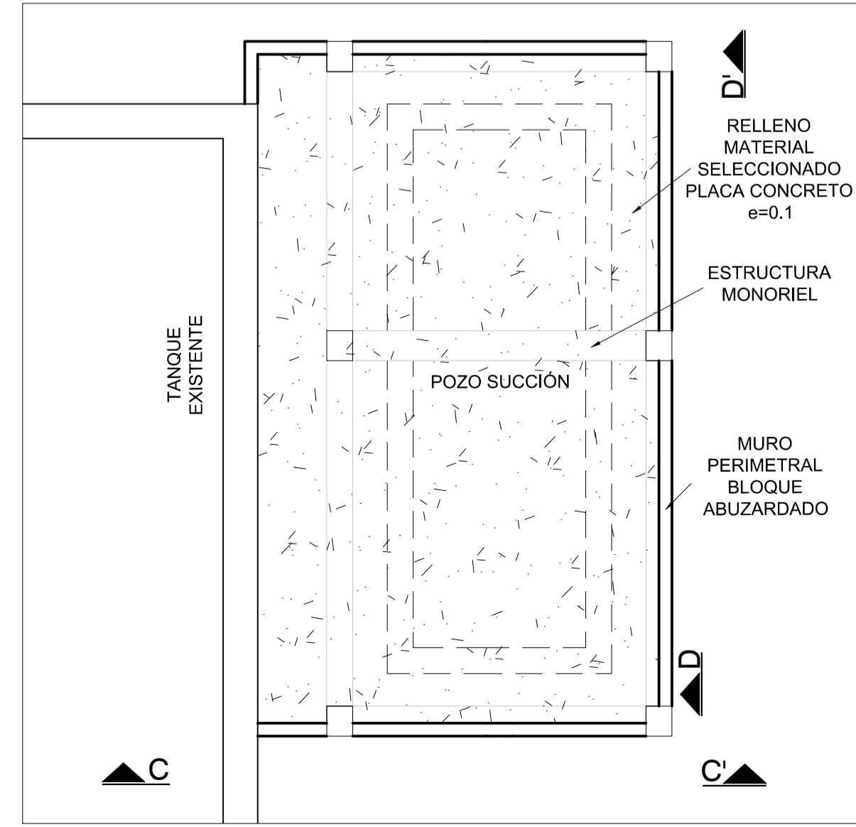
PLANTA MURO PERIMETRAL ESTRUCTURAL MONORIEL ESC. 5/E
