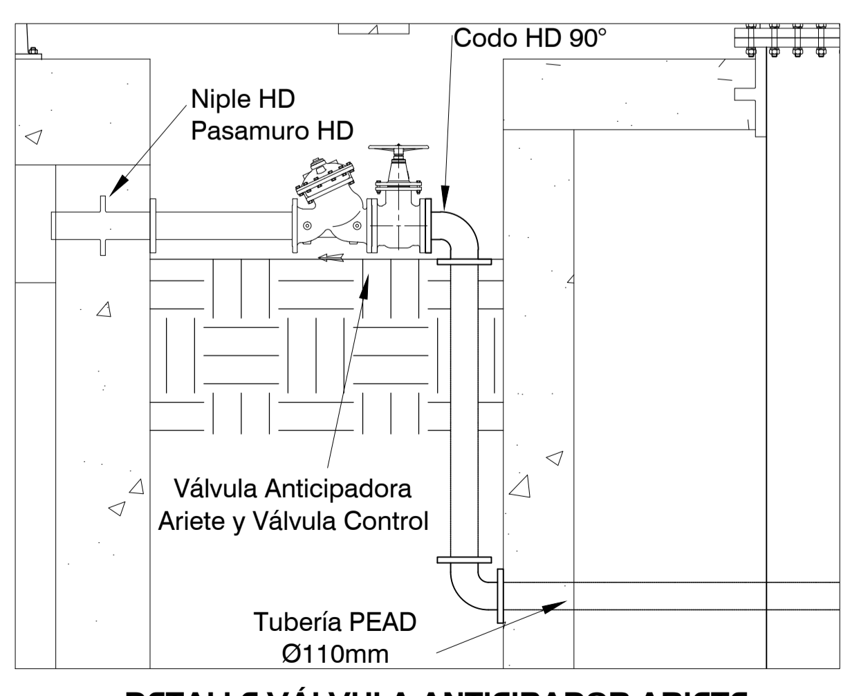
DETALLE VÁLVULA ANTICIPADOR ARIETE ESC. 5/E
