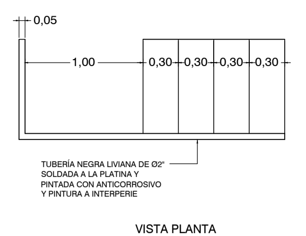
VISTA PLANTA
