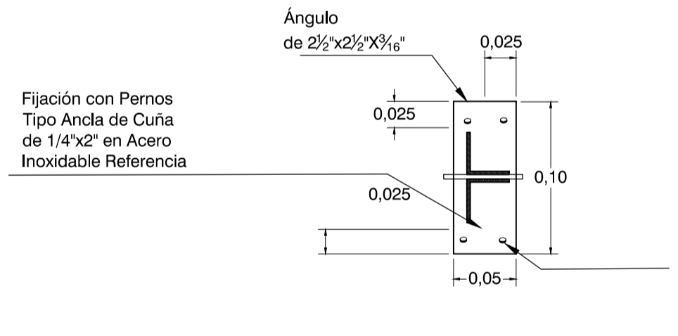
DETALLE PLACA METALICA SOPORTE PLACAS PRFV ESC. 5/E
