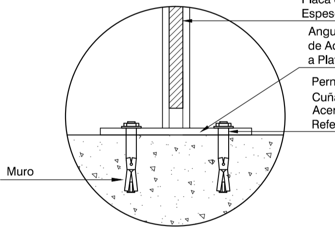
FIJACION DE PLATINA EN LOSA DE FONDO ESC. 5/E
