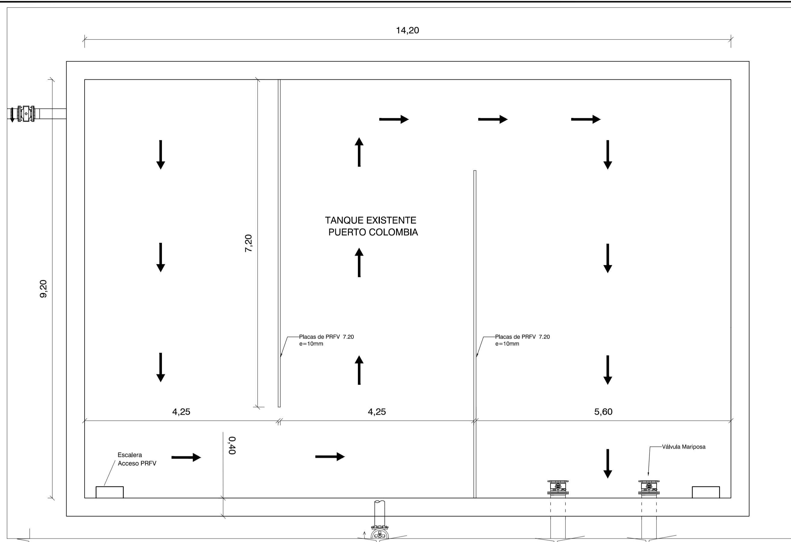
VISTA EN PLANTA TANQUE DE ALMACENAMIENTO EXISTENTE ESC. 5/E
