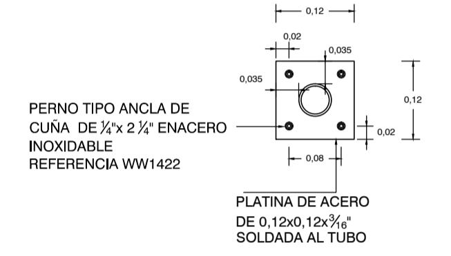
PERNO TIPO ANCLA DE CUÑA DE 1/2 x 2 1/2 EN ACERO INOXIDABLE REFERENCIA WW1422
