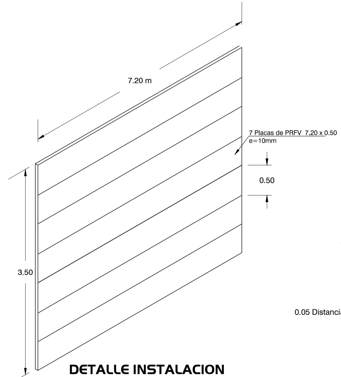
DETALLE INSTALACION PLACA TANQUE ESC. 5/E
