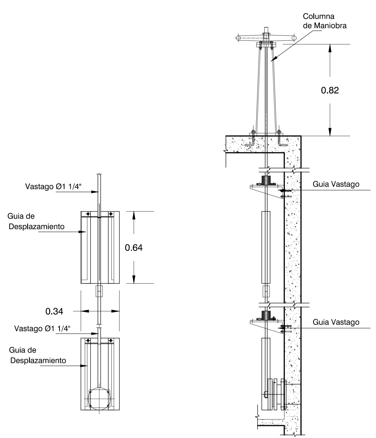
ENSAMBLE TÍPICO Y PERFIL DE MONTAJE DE VALVULA MARIPOSA
