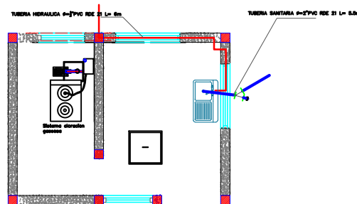
PLANTA HIDRAULICA CASETA OPERADOR CLORACION ESCALA 1:25
