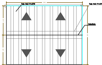
PLANTA DE CUBIERTA CASETA OPERADOR ESCALA 1:25
