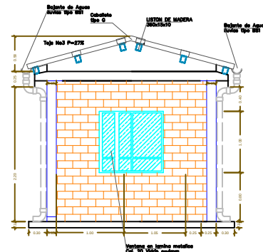
FACHADA LATERAL CASETA OPERADOR ESCALA 1:25
