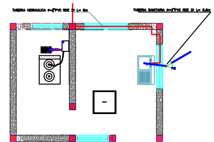
PLANTA SANITARIA CASETA OPERADOR CLORACION ESCALA 1:25
