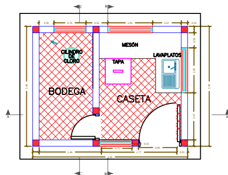
PLANTA ARQUITECTONICA CASETA OPERADOR ESCALA 1:25
