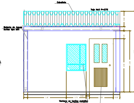
FACHADA PRINCIPAL CASETA OPERADOR ESCALA 1:25
