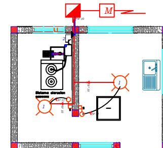
PLANTA ELECTRICA CASETA OPERADOR CLORACION ESCALA 1:25
