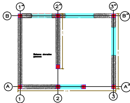
PLANTA ESTRUCTURAL CASETA OPERADOR CLORACION ESCALA 1:25
