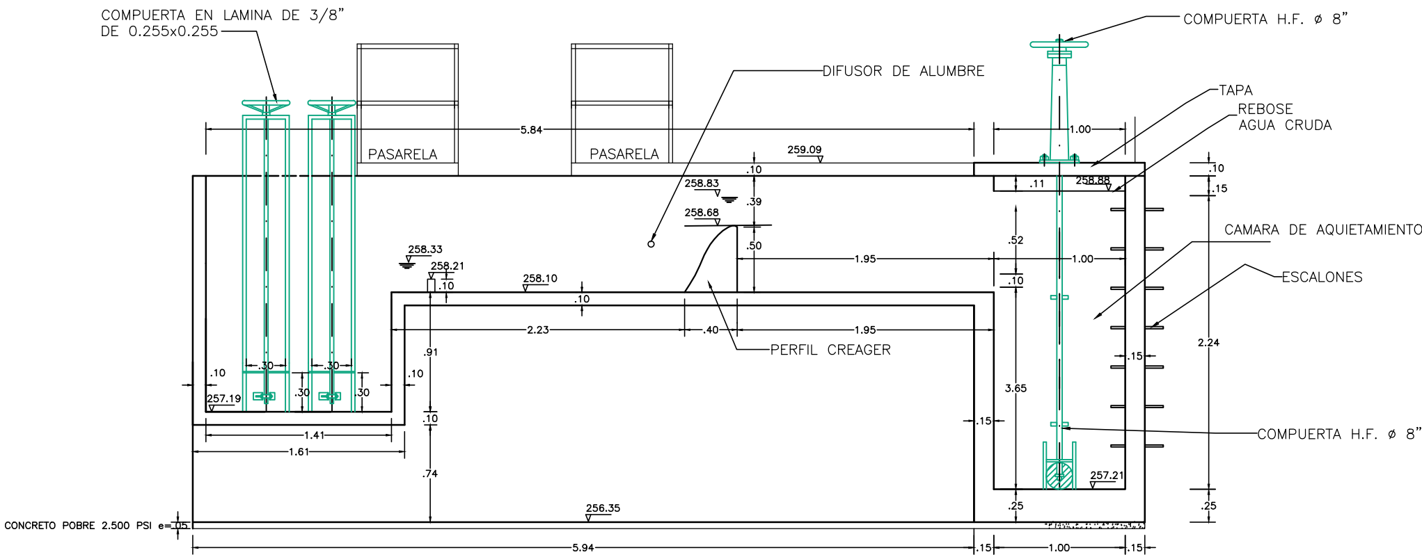
CORTE B-B
