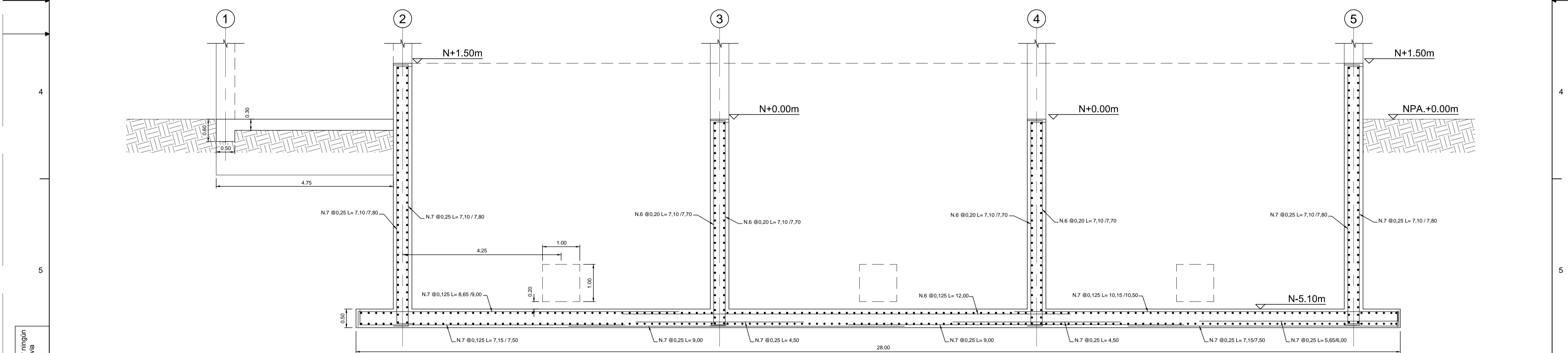
SECCIÓN C-C REFUERZO ESCALA 1:50
