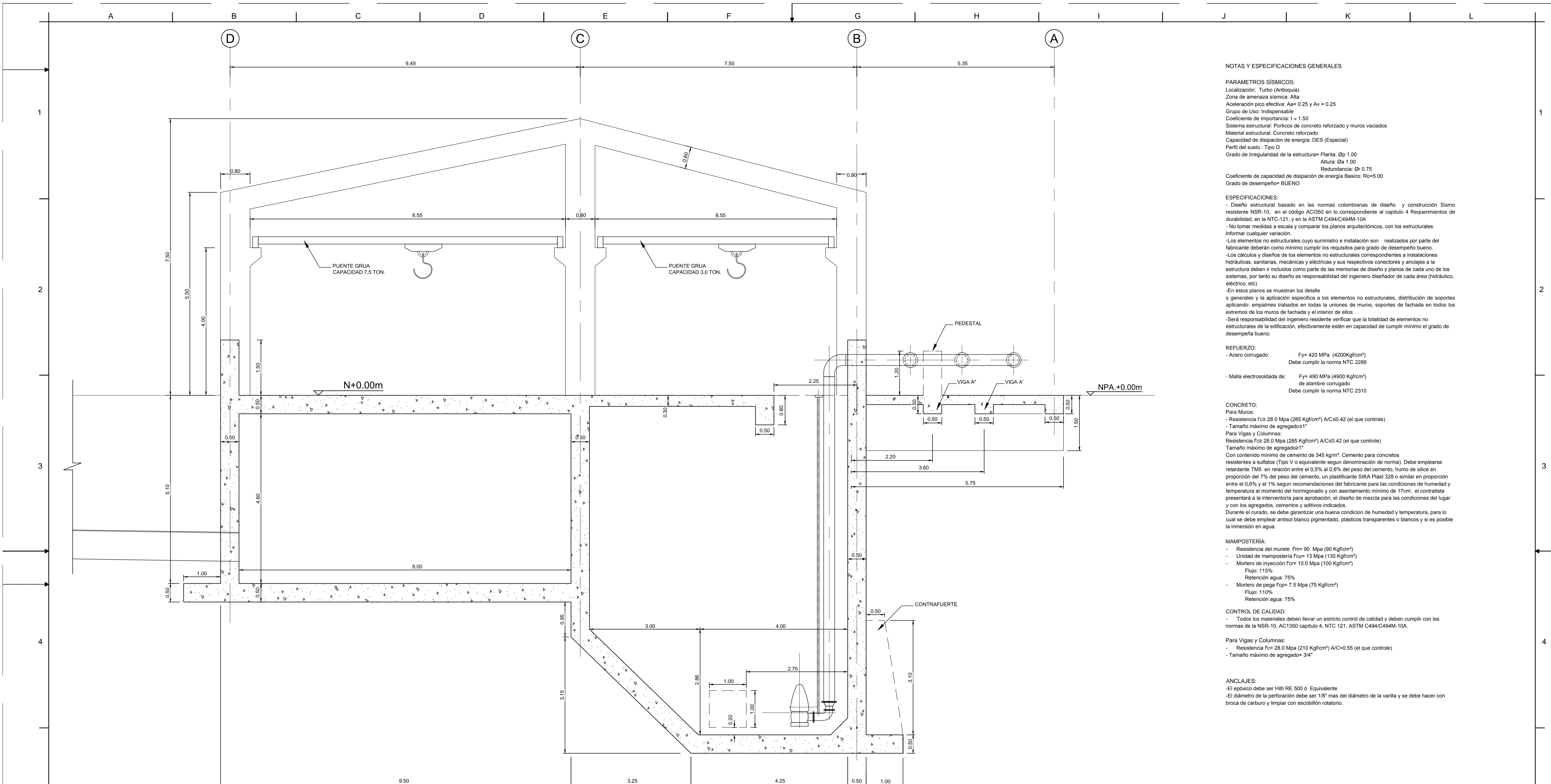
SECCIÓN D-D GEOMETRÍA ESCALA 1:50
