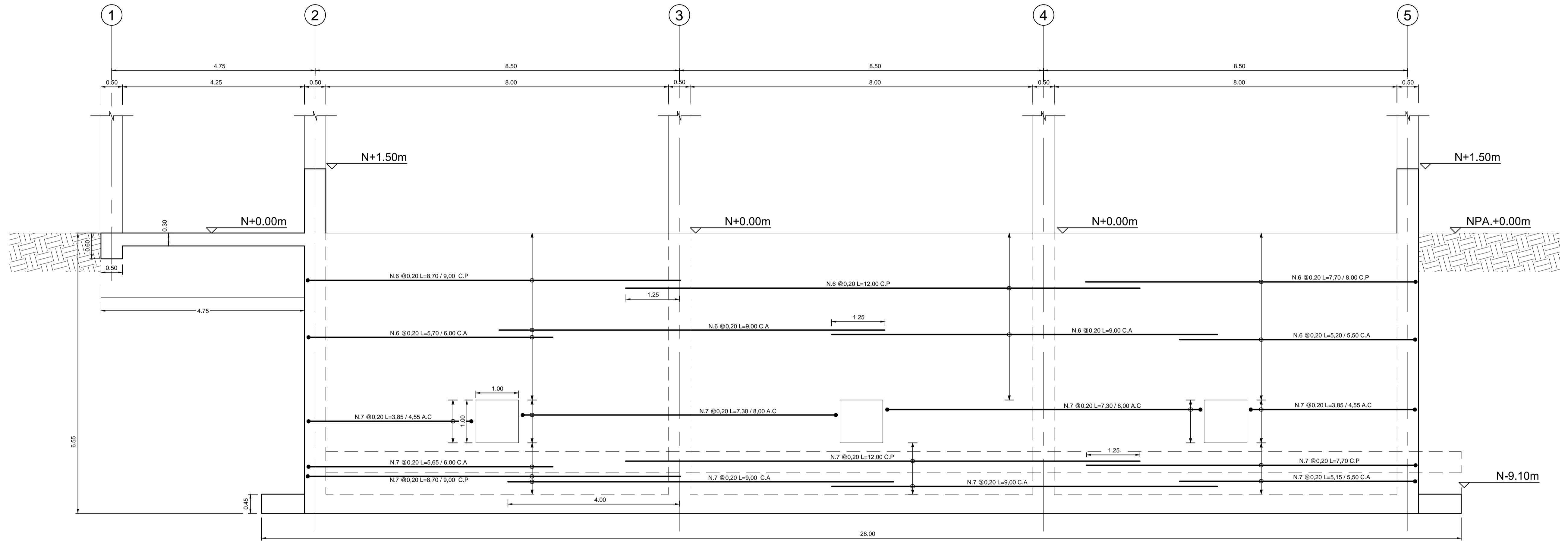
SECCIÓN POR EJE C REFUERZO HORIZONTAL EN MUROS ESCALA 1:50
