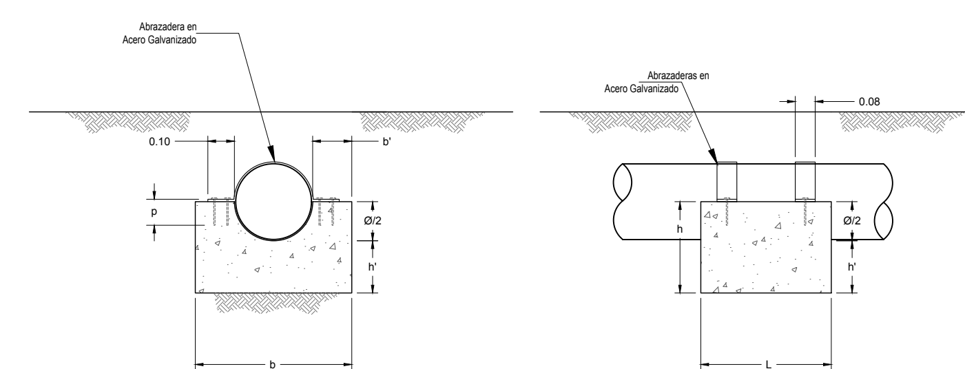
ESQUEMA DE ANCLAJES DE CURVA VERTICAL INFERIOR(EMPUJE HACIA ABAJO)
