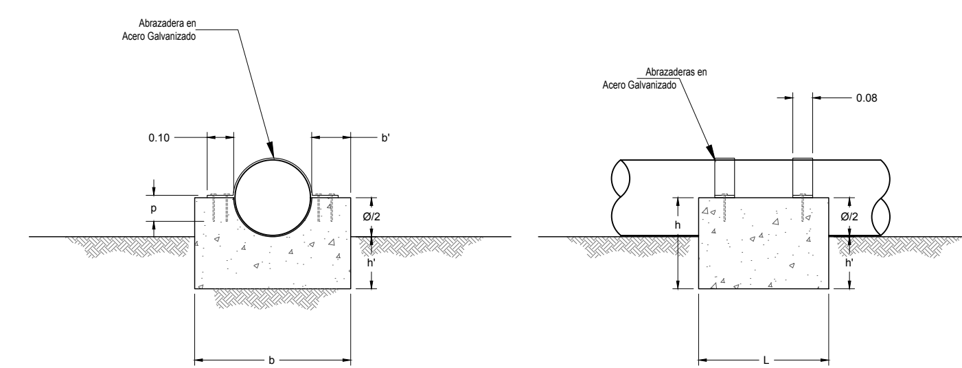
ESQUEMA DE ANCLAJES DE CURVA VERTICAL SUPERIOR(EMPUJE HACIA ARRIBA)
