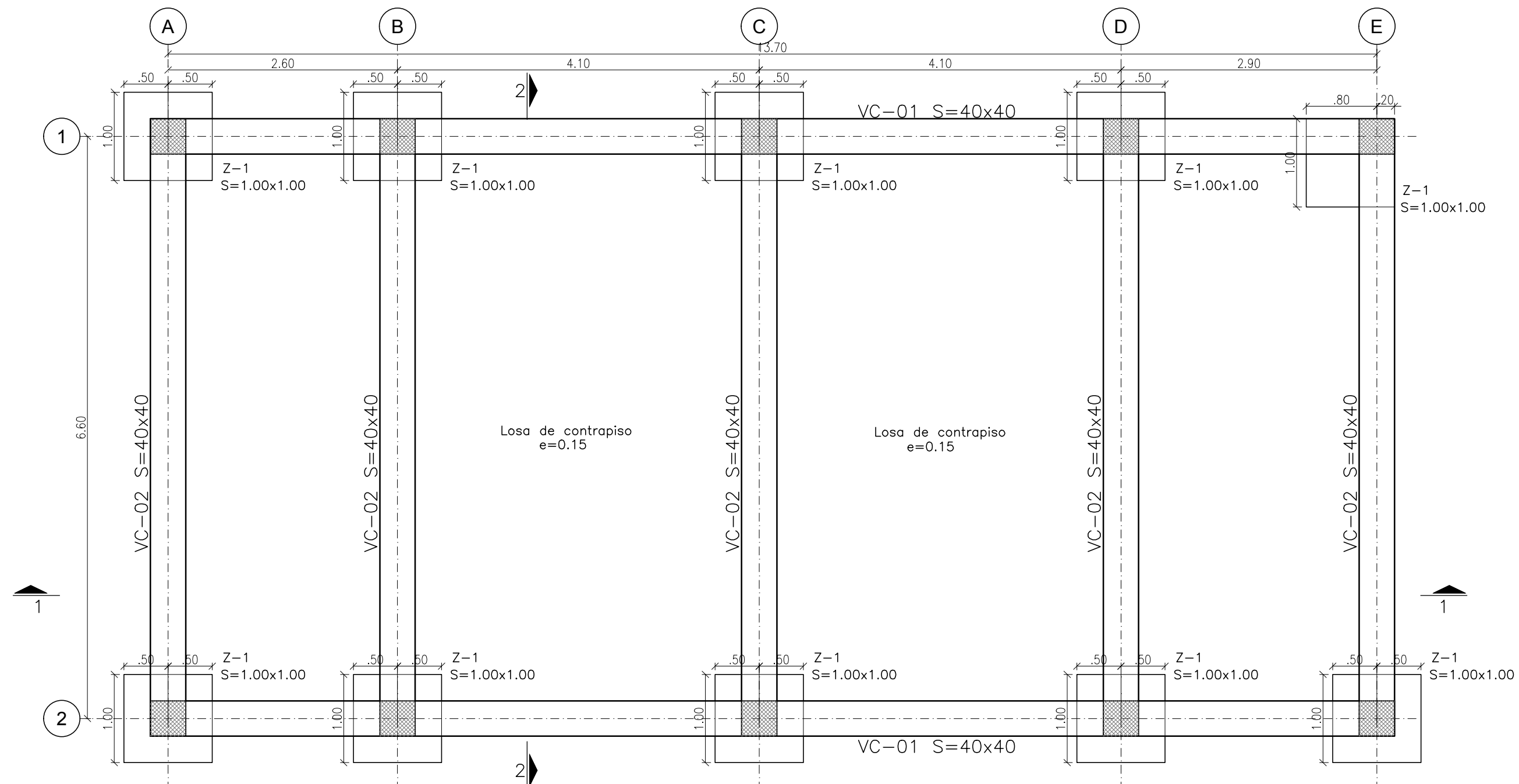
PLANTA CIMENTACIÓN ESCALA 1:50
