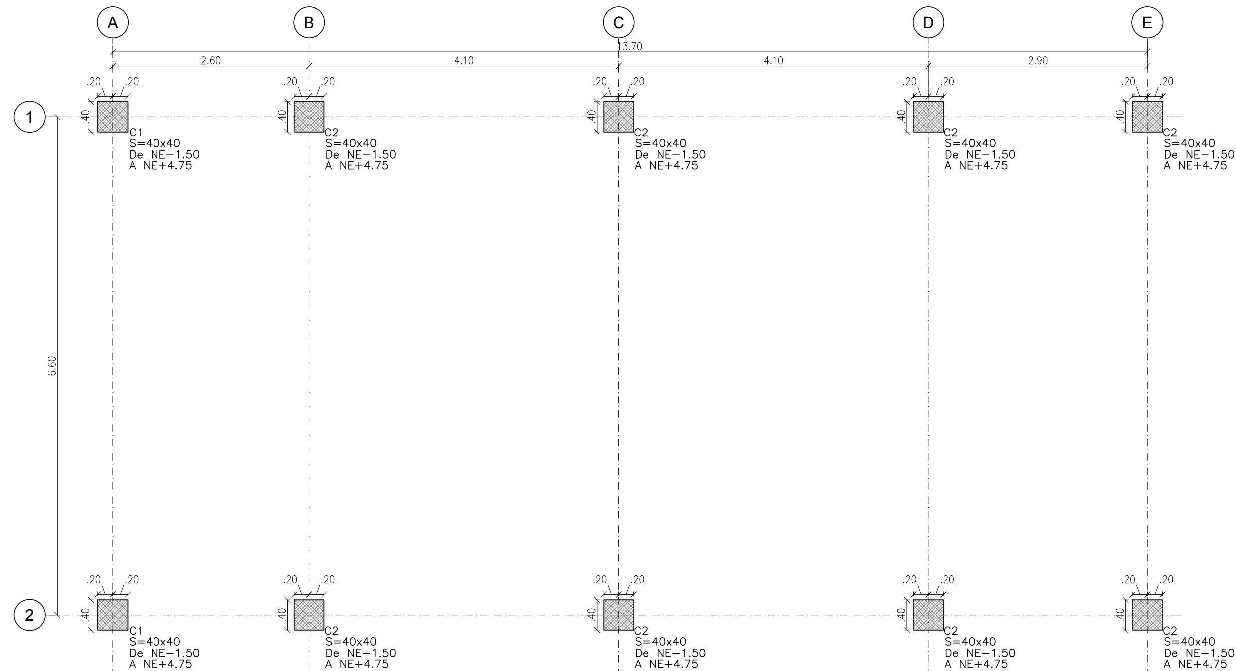
LOCALIZACIÓN DE COLUMNAS ESCALA 1:50
