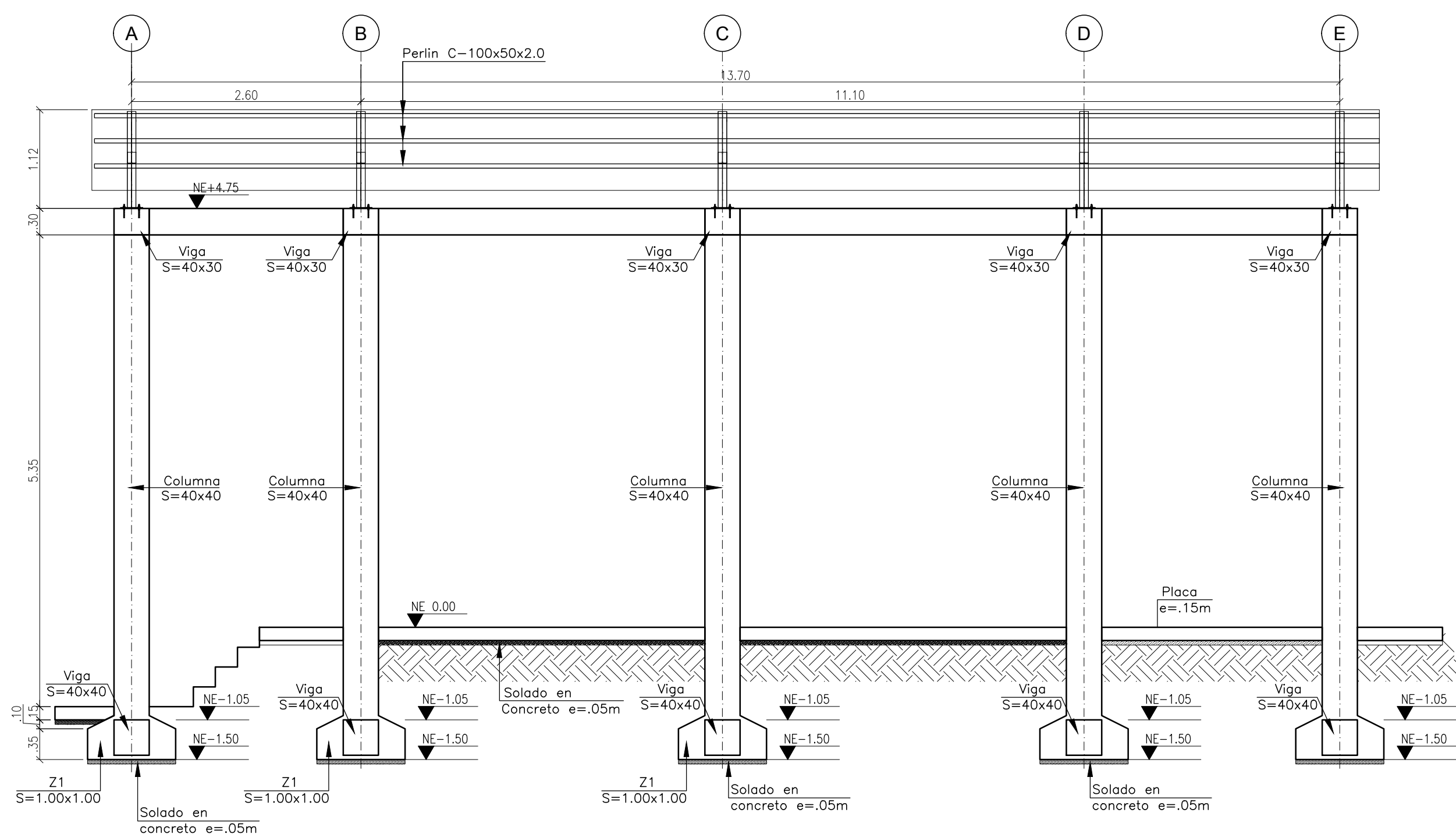
CORTE 1-1 ESCALA 1:50
