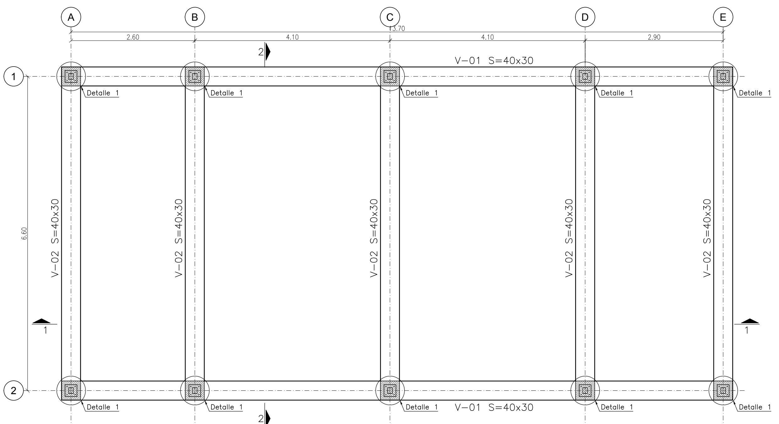
PLANTA VIGAS CUBIERTA ESCALA 1:50
