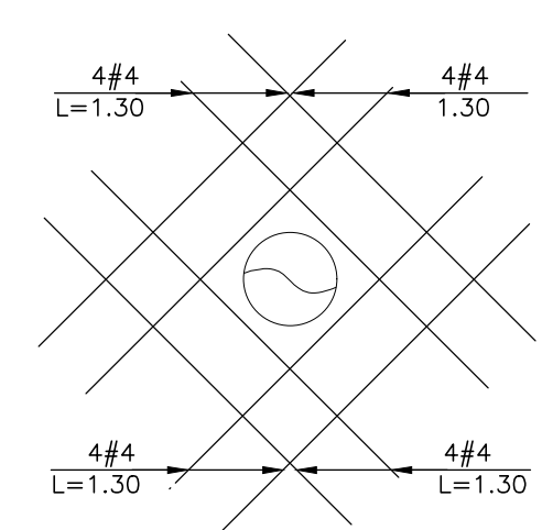
REFUERZO ADICIONAL HUECO TUBERIA ESCALA 1:25
