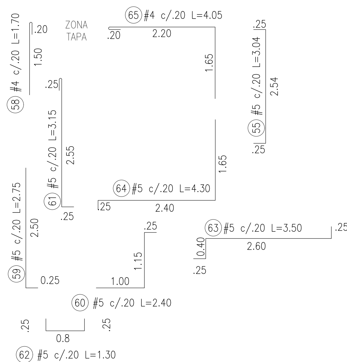
REFUERZO CORTE D-D ESCALA 1:50
