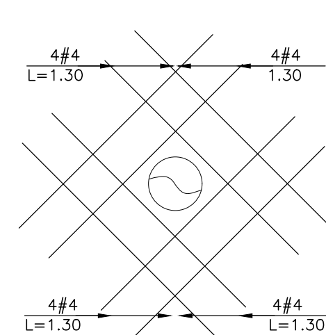
REFUERZO ADICIONAL HUECO TUBERIA ESCALA 1:25
