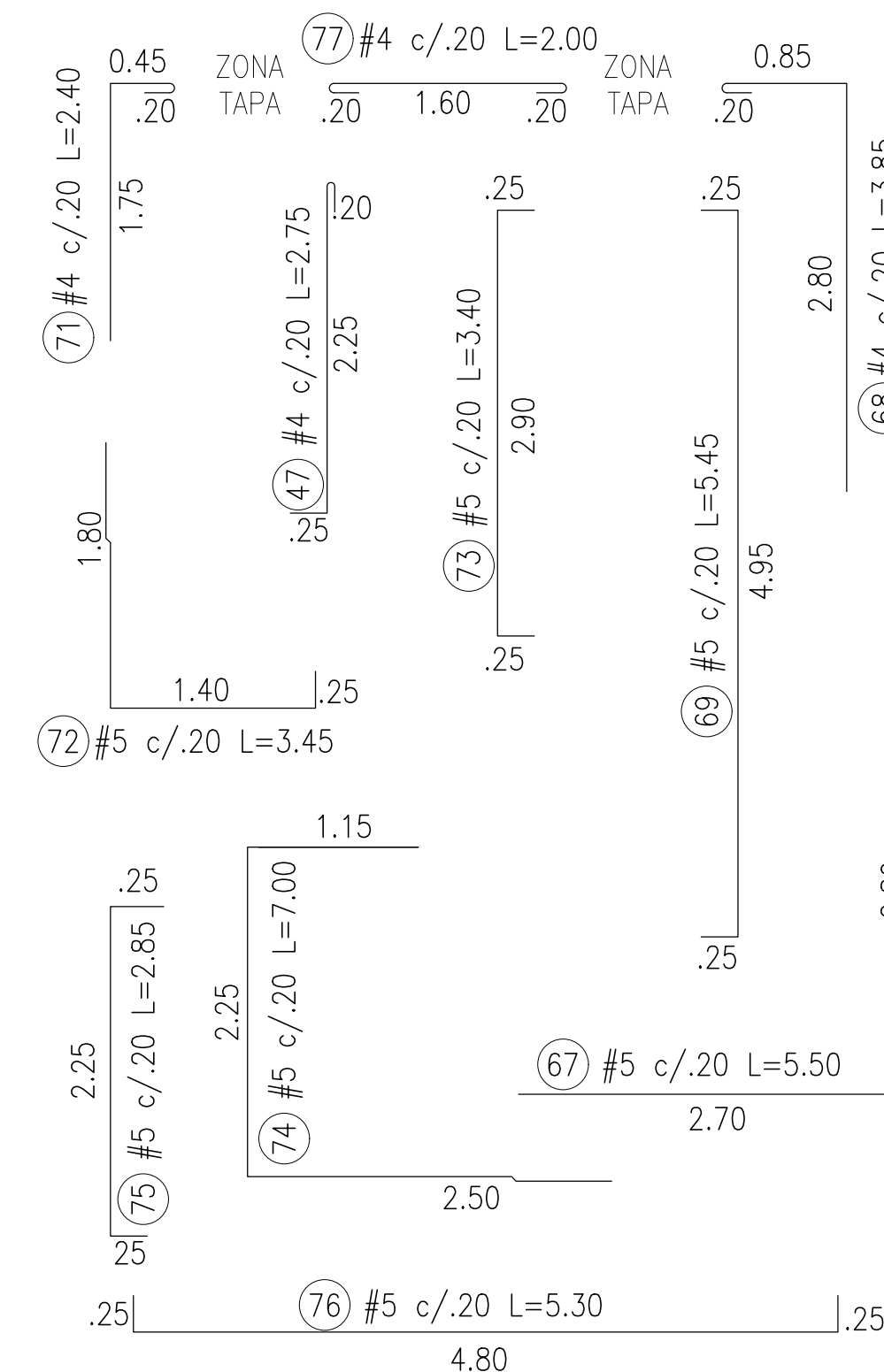
REFUERZO CORTE F-F ESCALA 1:50
