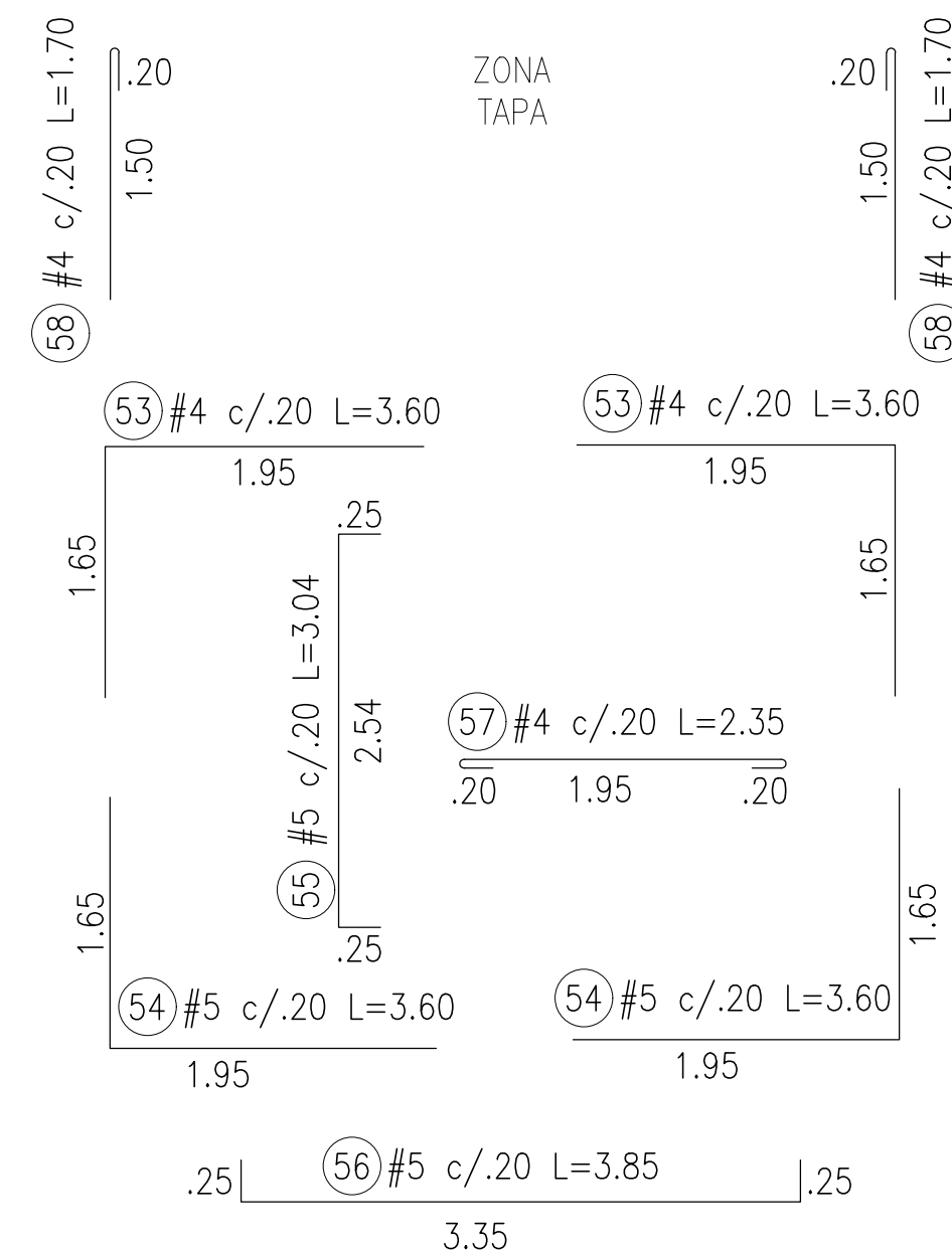
REFUERZO CORTE C-C ESCALA 1:50
