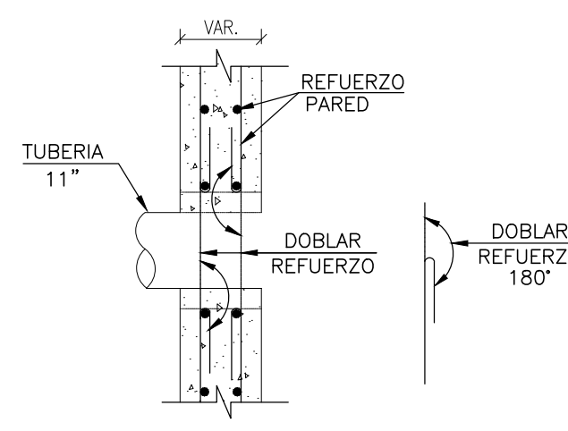
HUECO TUBERIA ALZADO O PLANTA ESCALA 1:25
