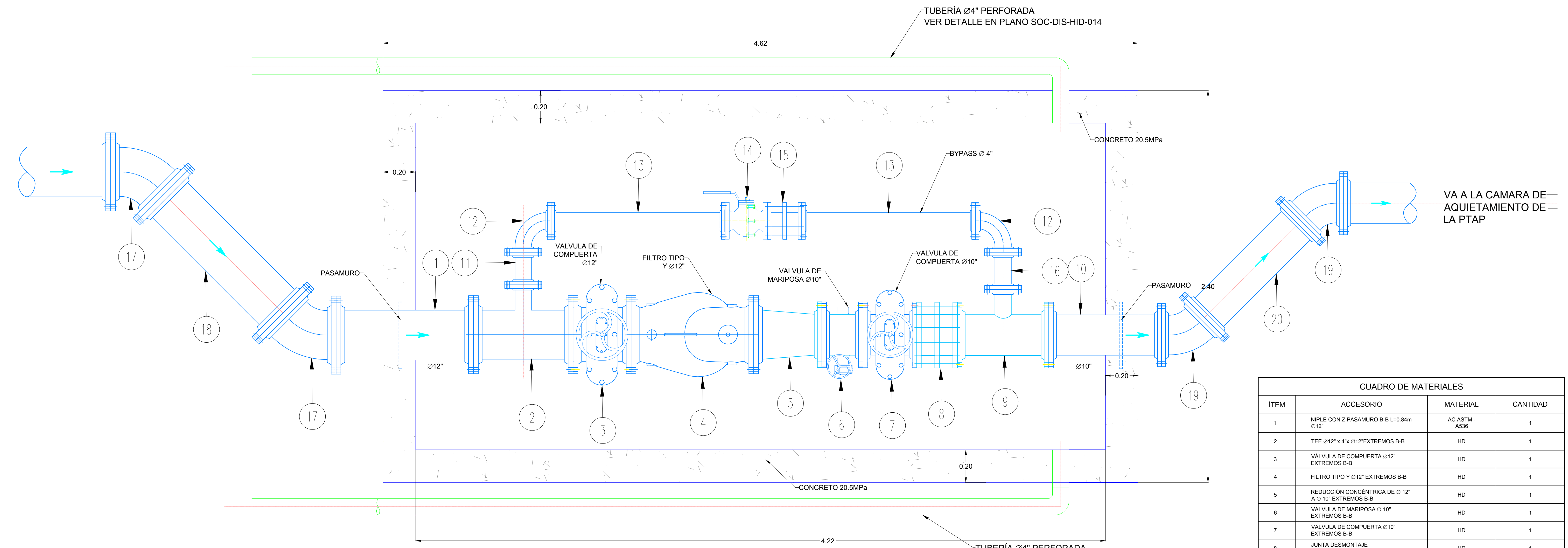
PLANTA CÁMARA DE VÁLVULAS ENTRADA VRP PTAP ESC: 1:10
