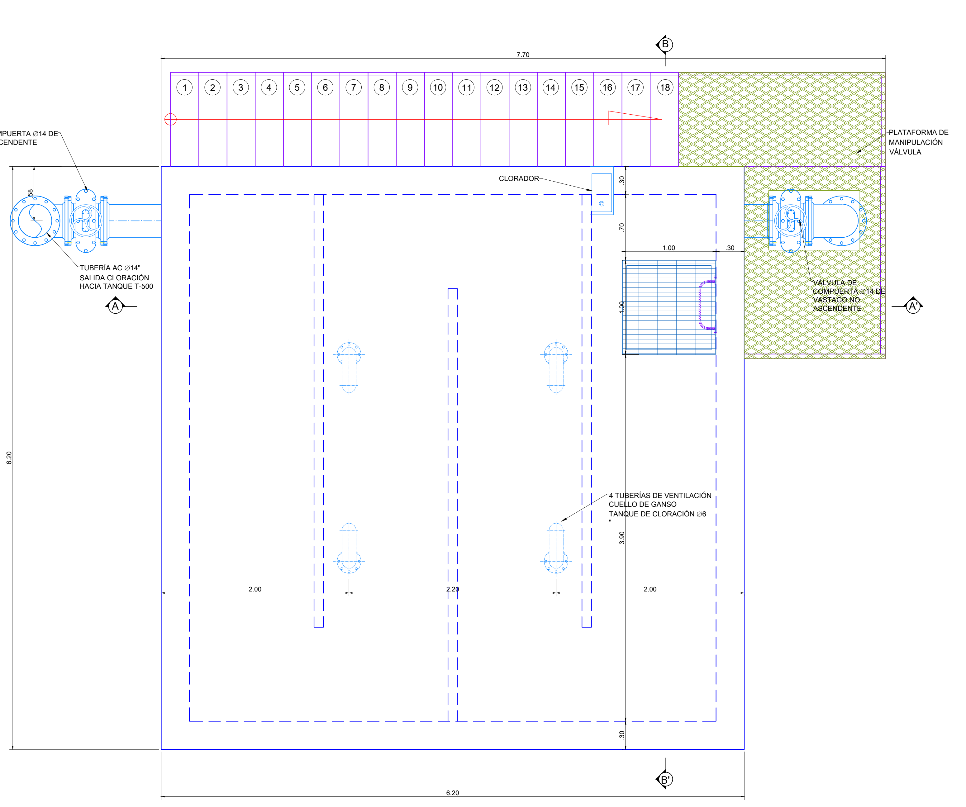
PLANTA TANQUE DE CLORACIÓN ESC: 1:25
