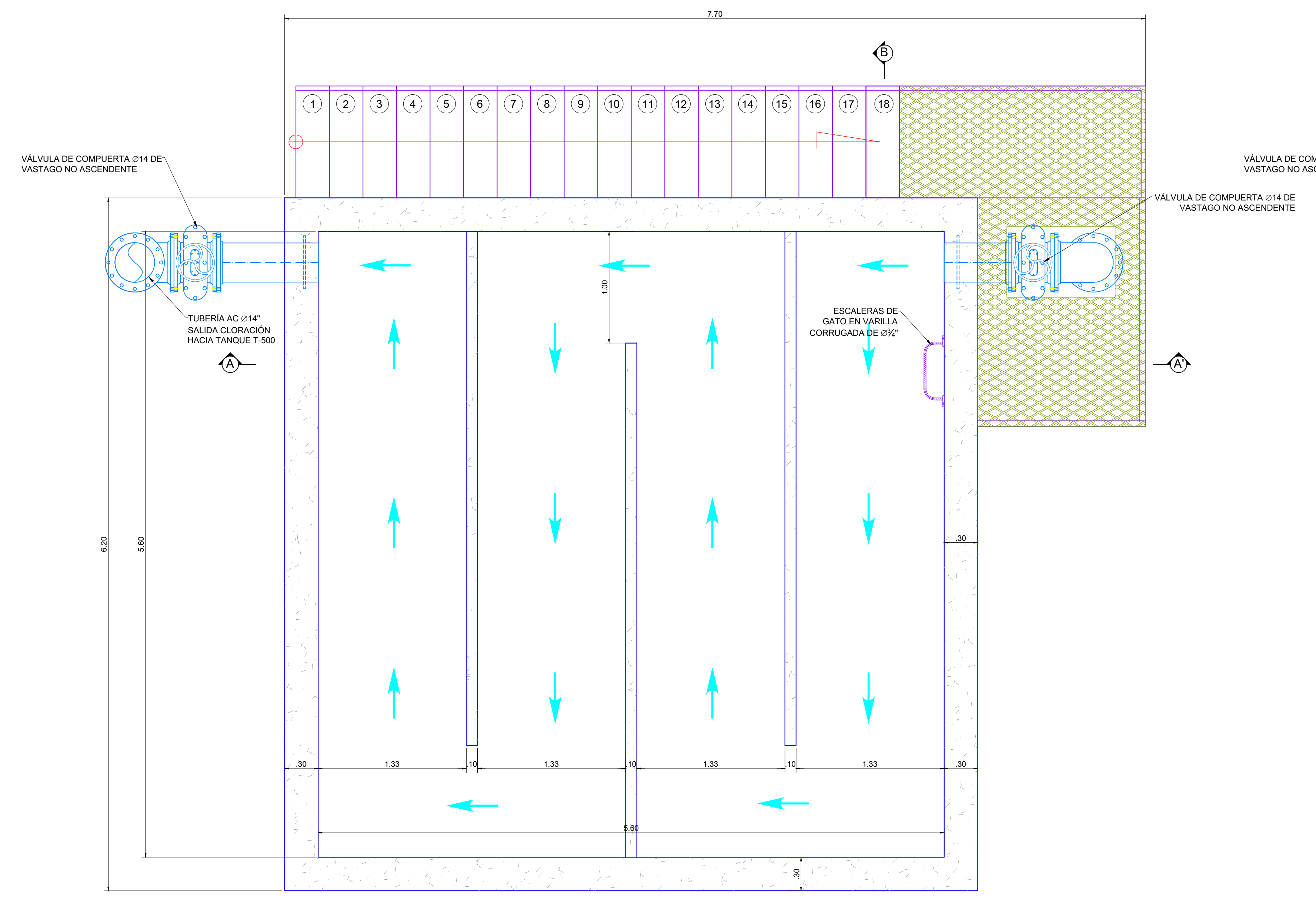
CORTE PLANTA 1-1' TANQUE DE CLORACIÓN ESC: 1:25
