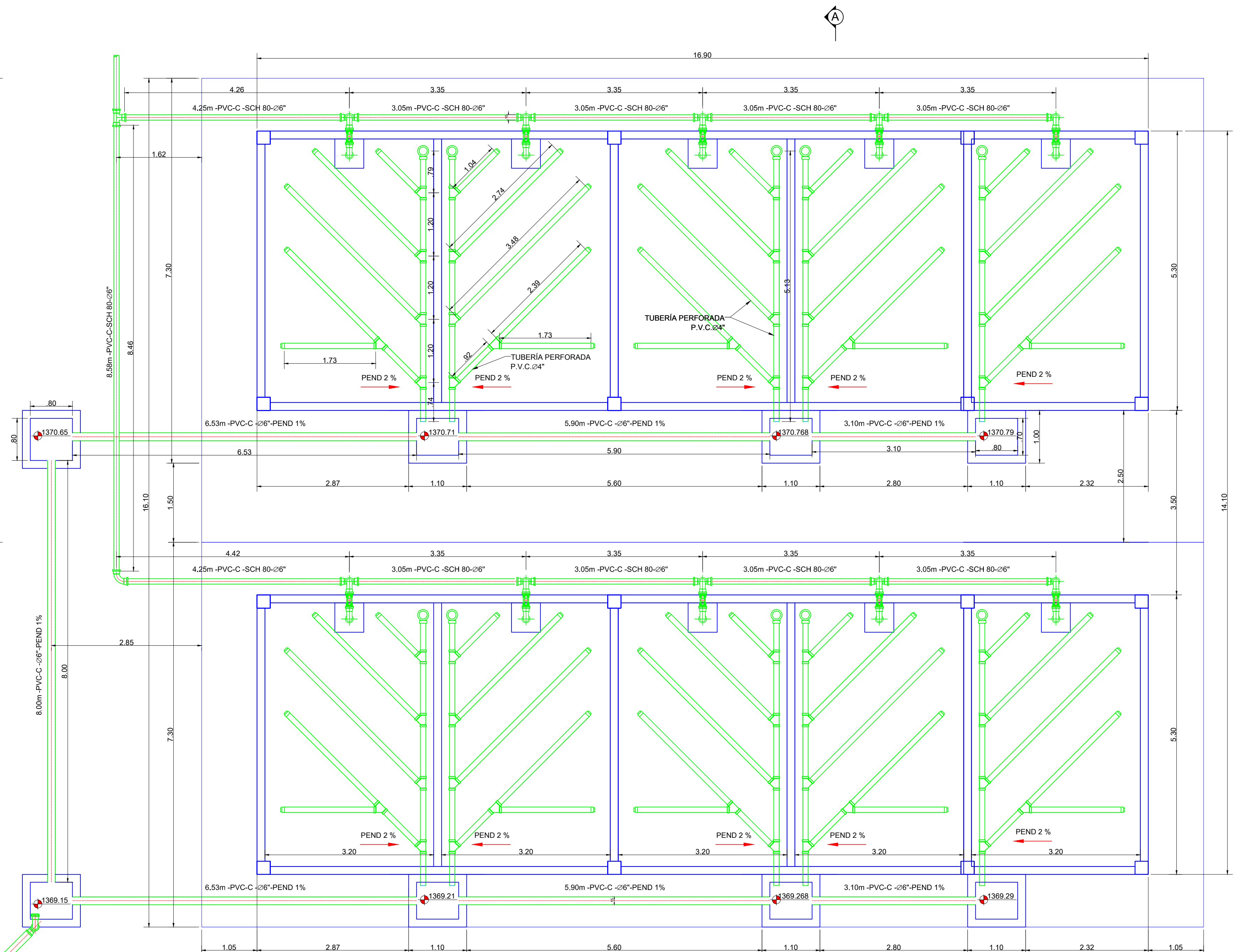
PLANTA LECHOS DE SECADO ESC: 1:50
