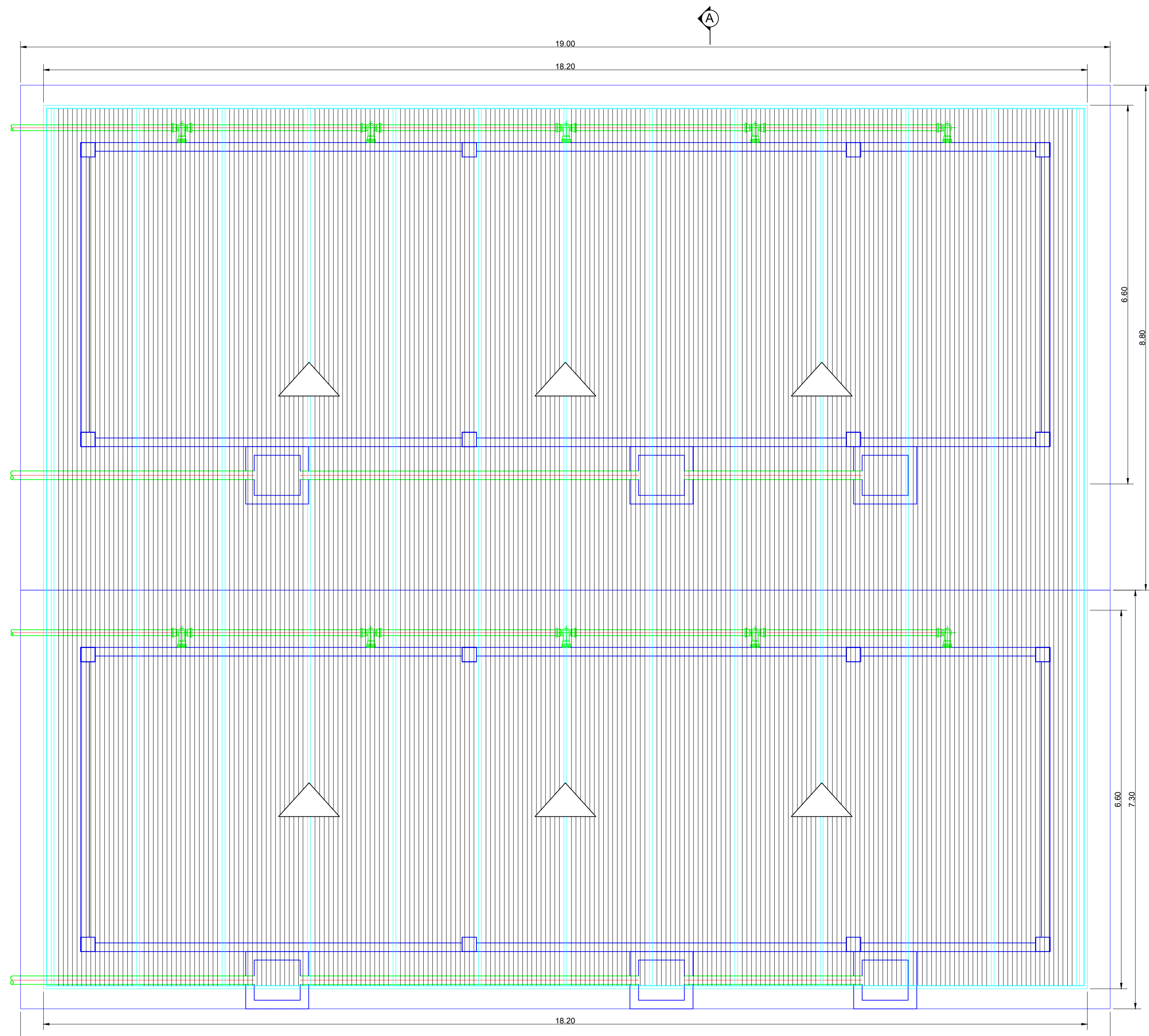
PLANTA DE CUBIERTAS LECHOS DE SECADO ESC: 1:50
