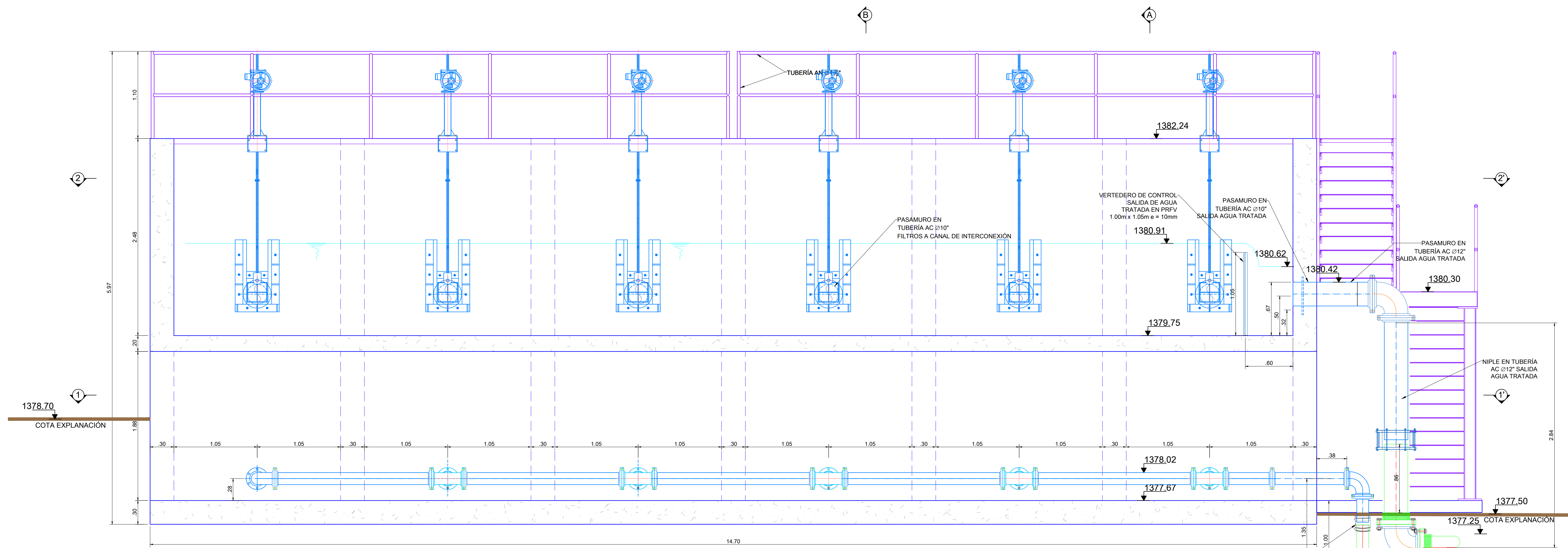
CORTE C-C' ESC. 1:25
