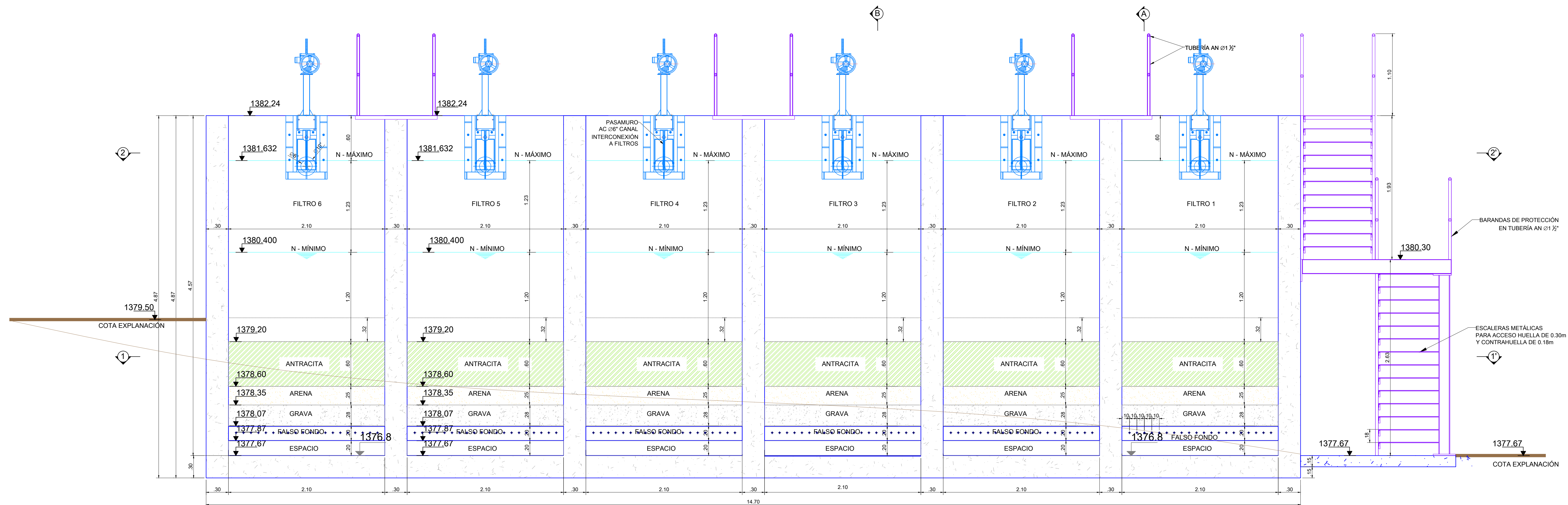
CORTE D-D' ESC. 1:25
