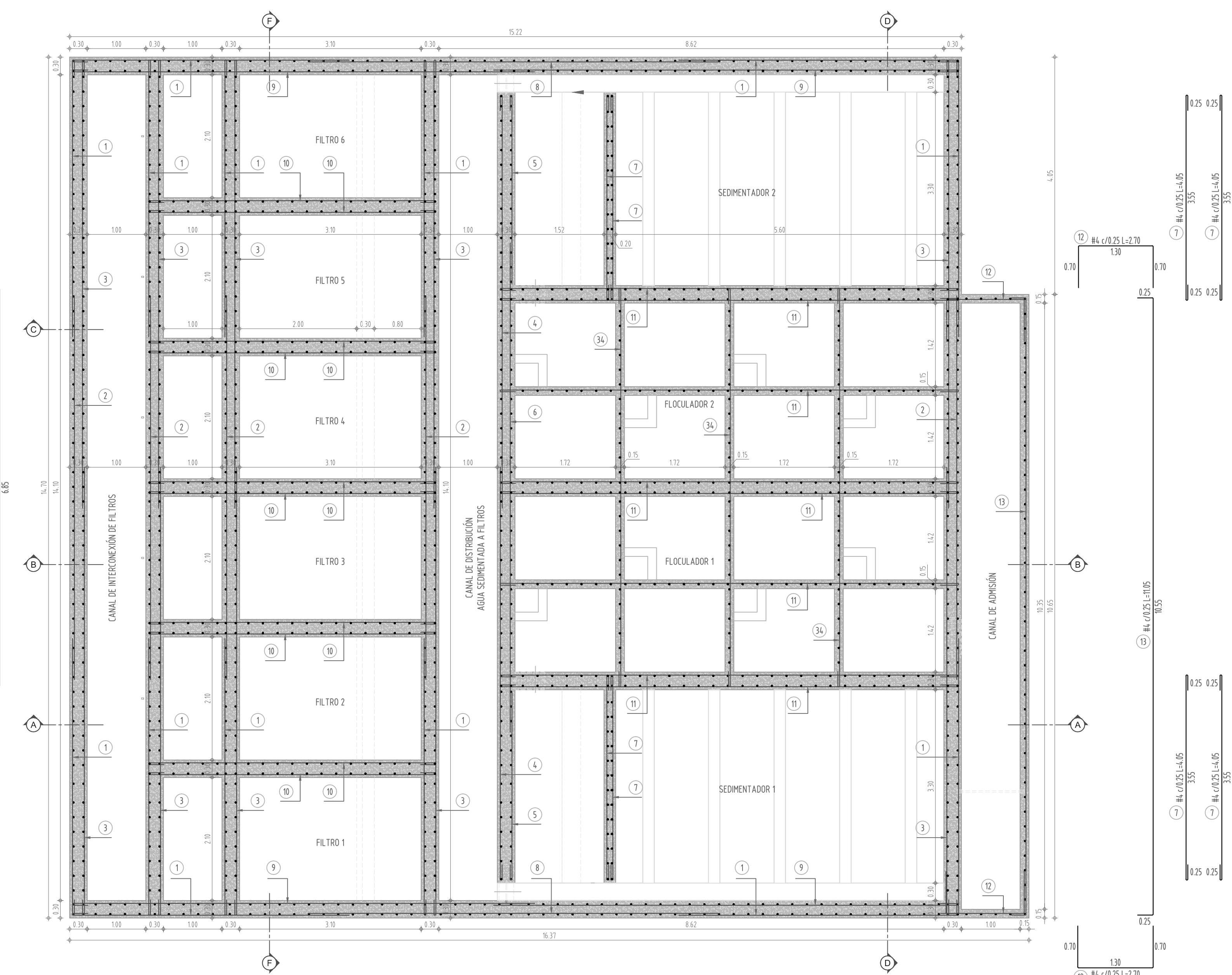
CORTE 2-2 PLANTA ESTRUCTURAL NIVEL POR DEBAJO DE PASARELAS PLANTA DE TRATAMIENTO Escala: 1:50
