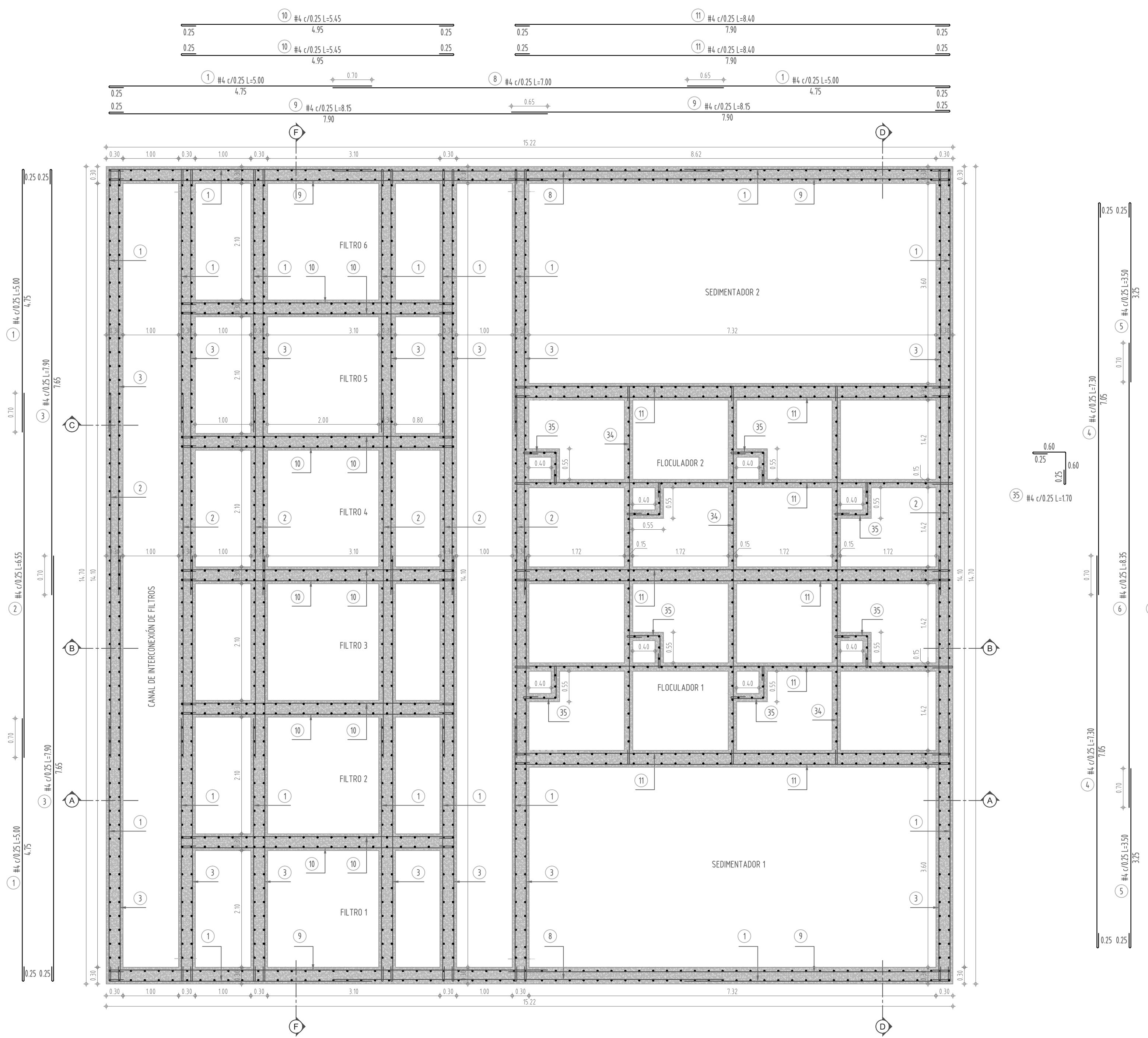
CORTE 1-1 PLANTA ESTRUCTURAL FONDO-DESAGÜES PLANTA DE TRATAMIENTO Escala: 1:50
