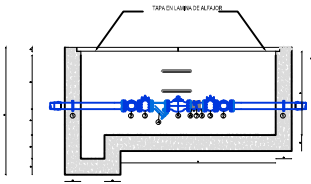
CORTE A-A DETALLES ESTACION REDUCTORA DE PRESIÓN ESC. 1:25
