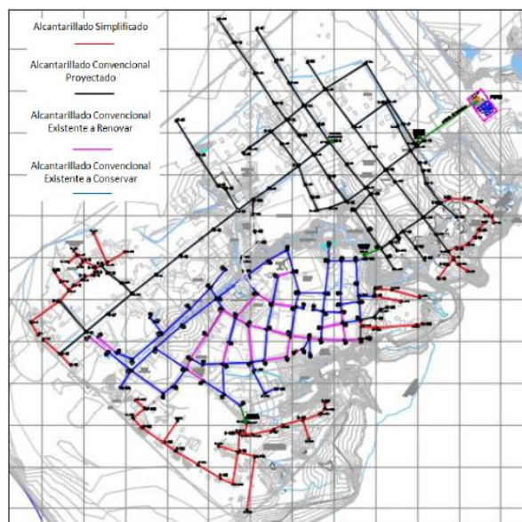
Fig. 4 Esquema General del sistema de alcantarillado de Bajo Baudó
