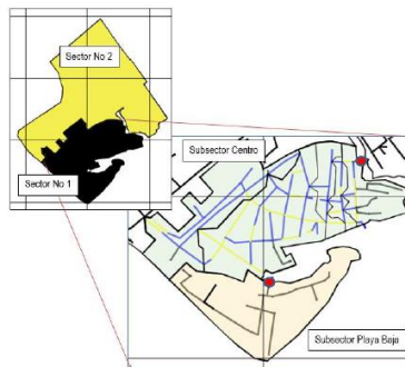
Fig. 2 Subdivisión Sector No. 1 Alcantarillado del Municipio
