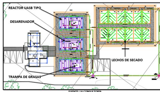
Fig. 7 Esquema general Planta de Tratamiento de Aguas Residuales
