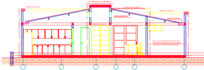
CORTE B'B' 1:50
