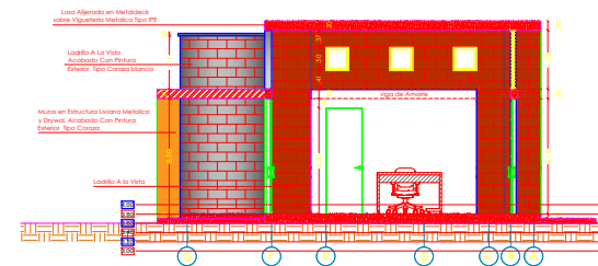
CORTE A'A' 1:50
