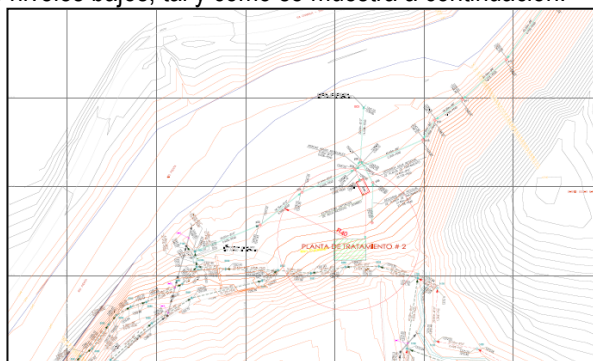
Ilustración 2 Plano Planta General – Conexión Alcantarillado A.R. a Planta de tratamiento #2
