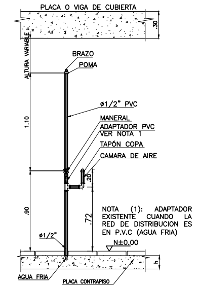
DETALLE 03 CONEXIONES A DUCHA CON GRIFERÍA ESTÁNDAR ESC 1:20
