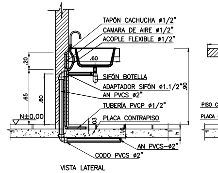
DETALLE 01 CONEXIONES LAVAPLATOS ESC 1:20
