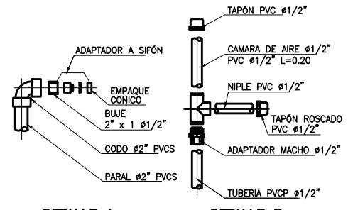
DETALLE A ESC SIN DETALLE B MONTAJE CAMARA DE AIRE PVC-AF ESC SIN
