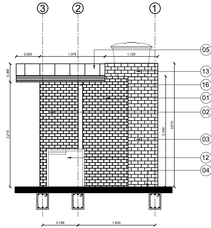
Fachada Sur
