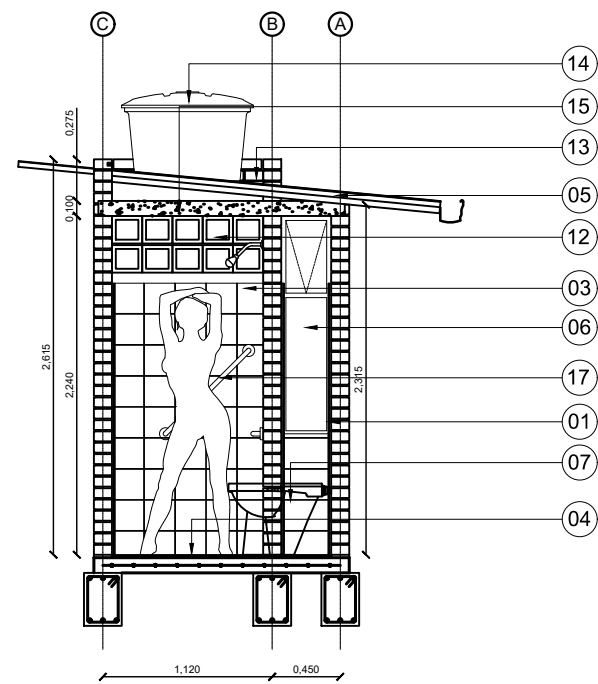
Sección B-B
