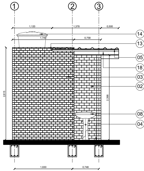
Fachada Norte
