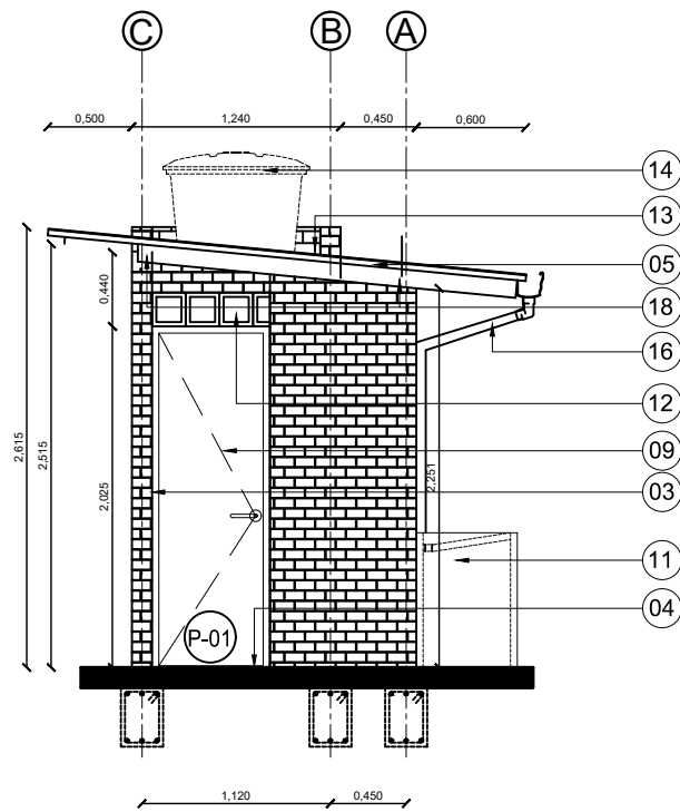
Fachada Occidental
