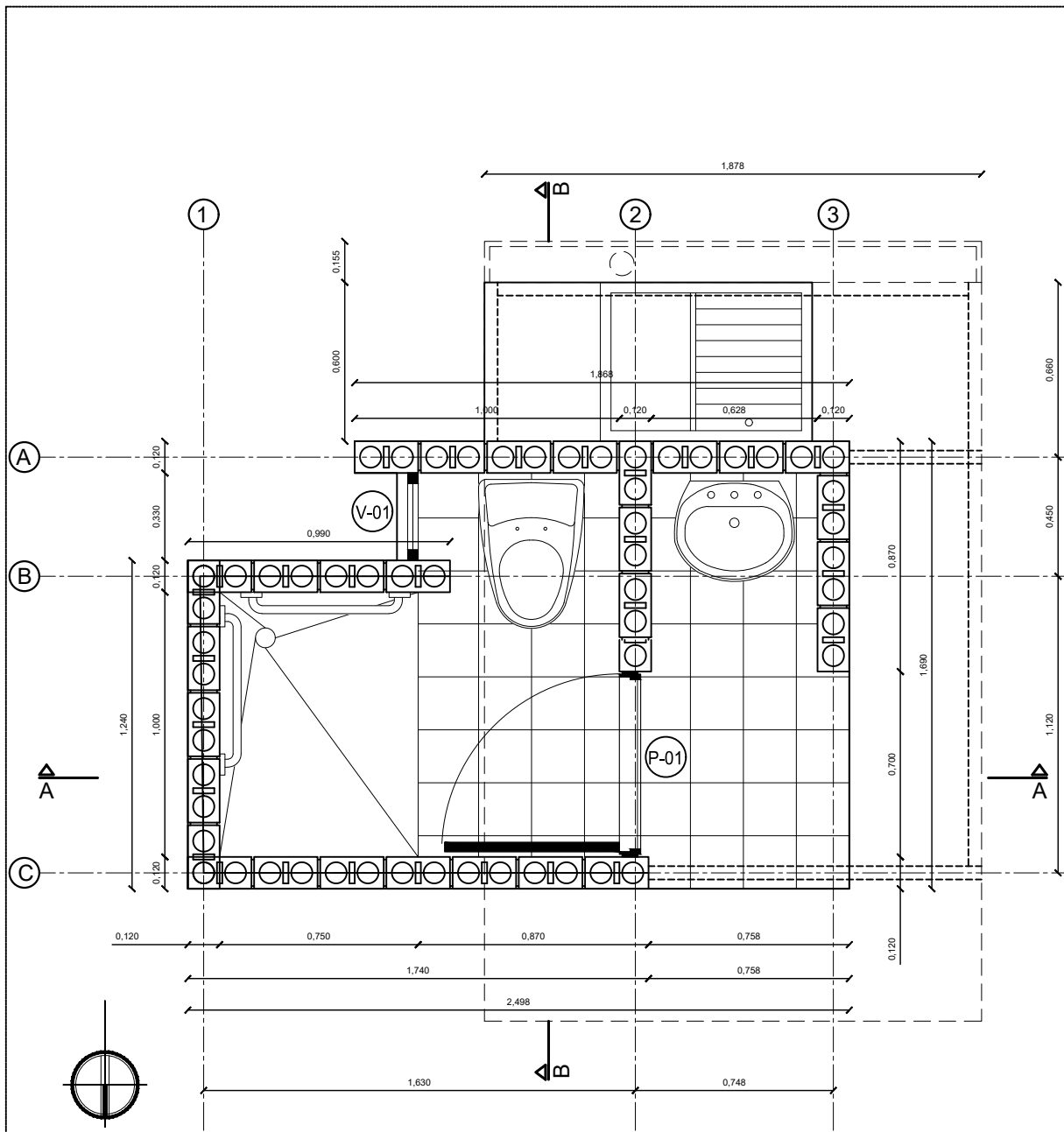
Planta
