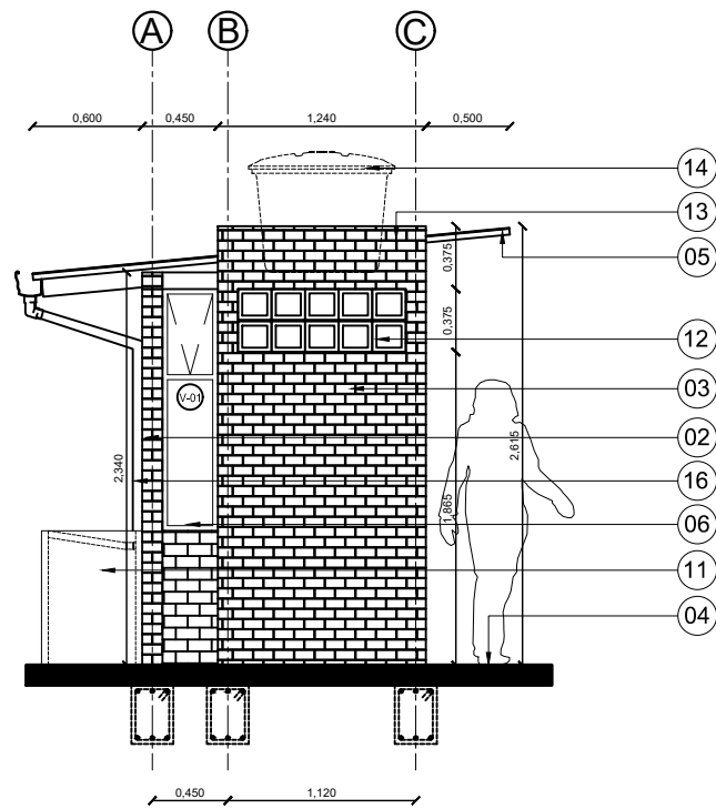
Fachada Oriental
