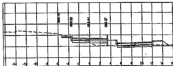
Sección típica doble calzada - par vial
