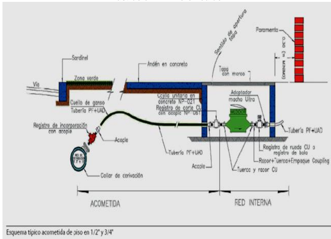
Ilustración 4-1 Micromedidor
