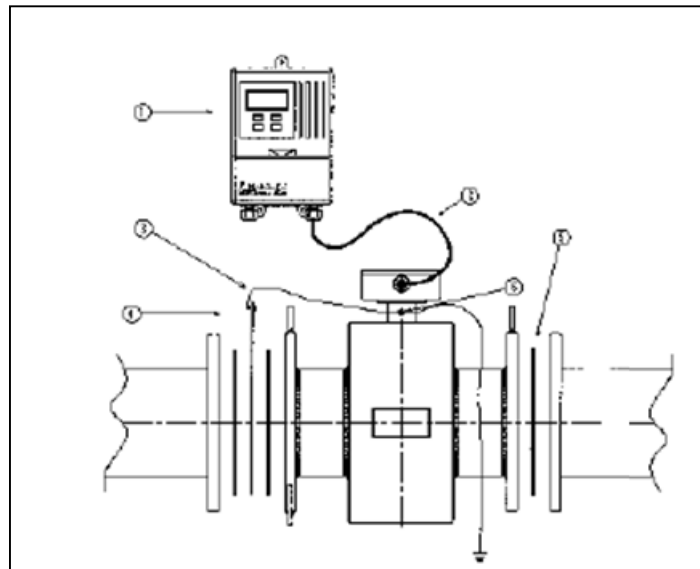
Ilustración 4-2 Macromedidor
