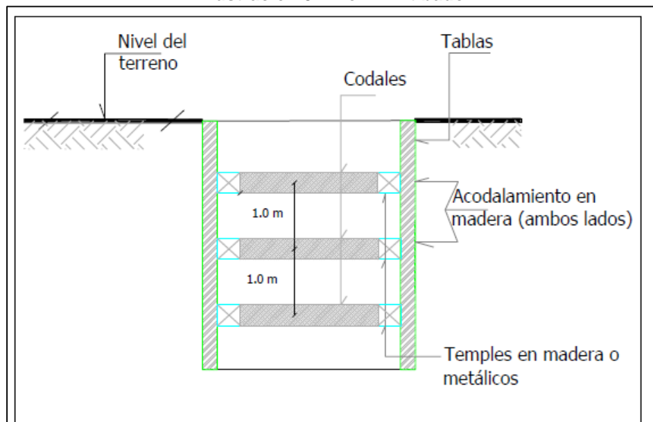
Ilustración 3-2 Perfil Entibado
