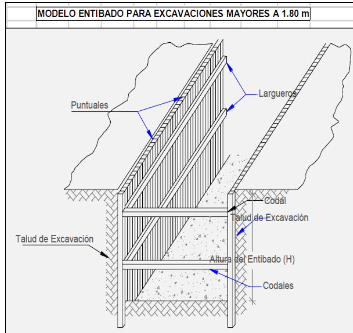
Ilustración 3-1 Entibados
