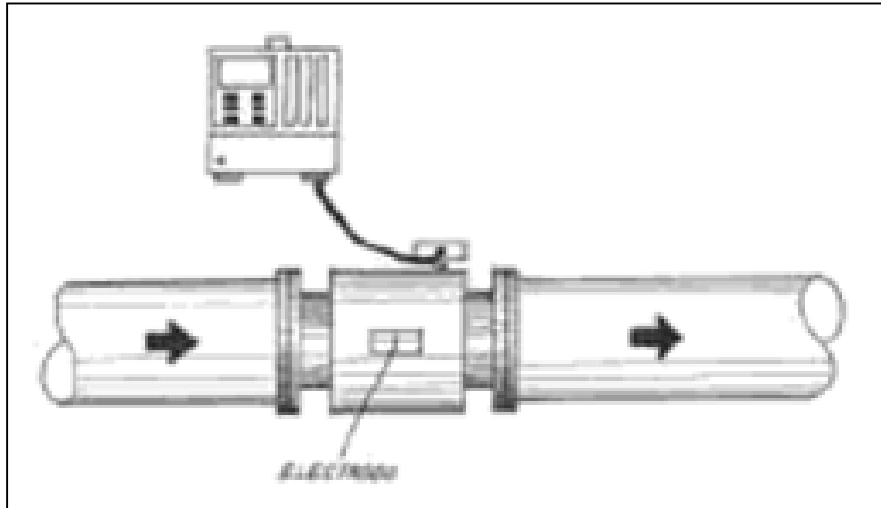
Ilustración 4-3 Macromedidor horizontal
