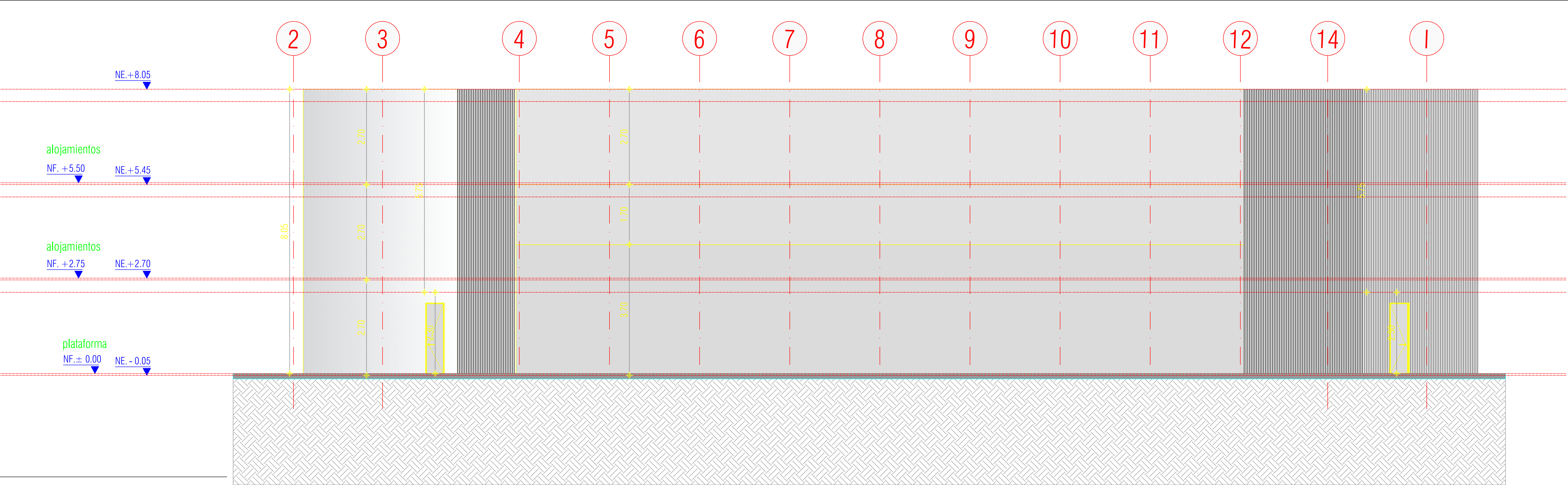
FACHADA SURESTE / BLOQUE H
